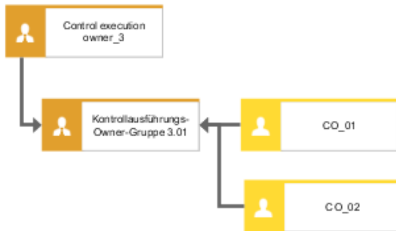
Abbildung 1: Struktur Benutzer/Benutzergruppen
