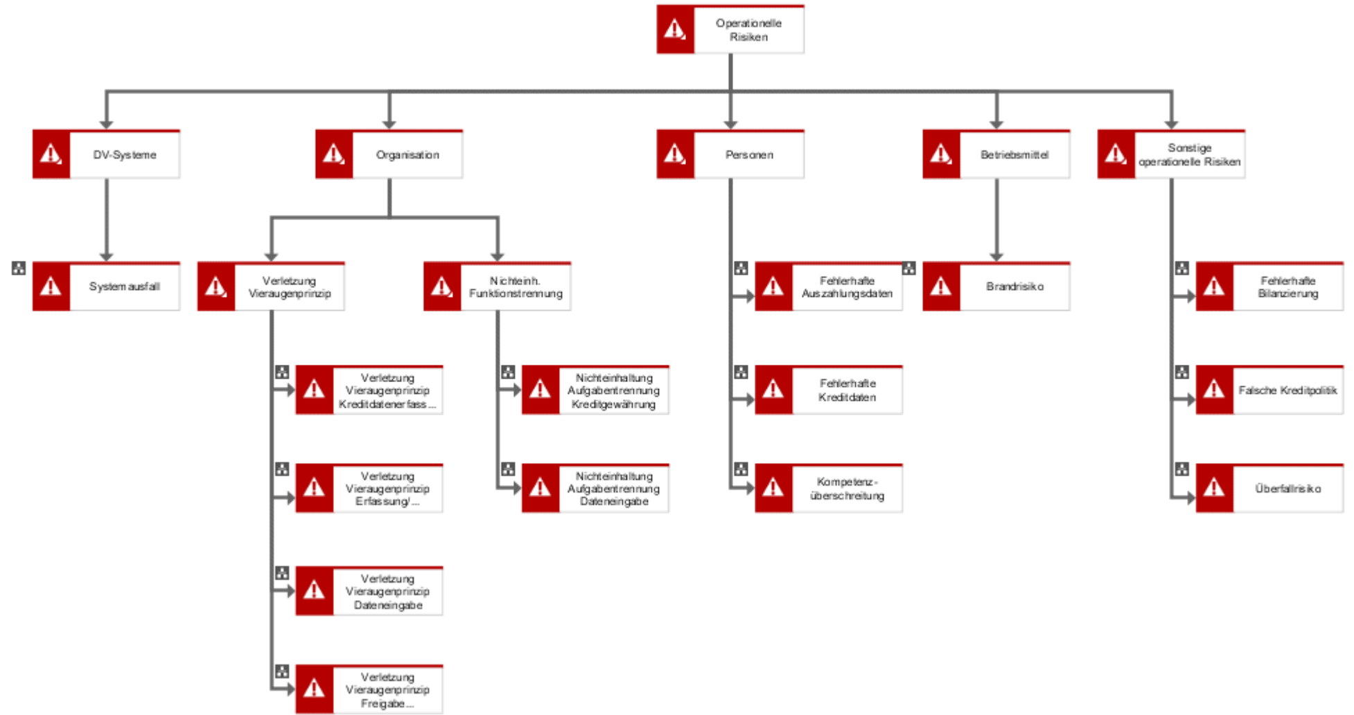
Abbildung 7: Struktur Risikohierarchie
