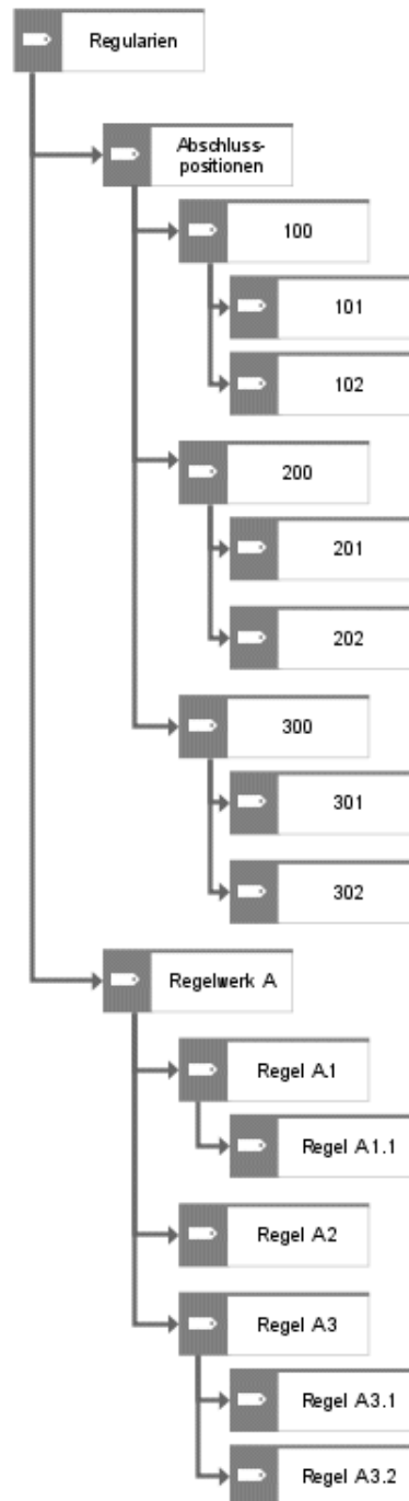
Abbildung 5: Struktur Regularienhierarchie
