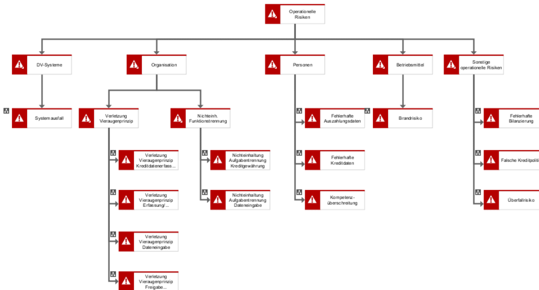
Abbildung 7: Struktur Risikohierarchie
