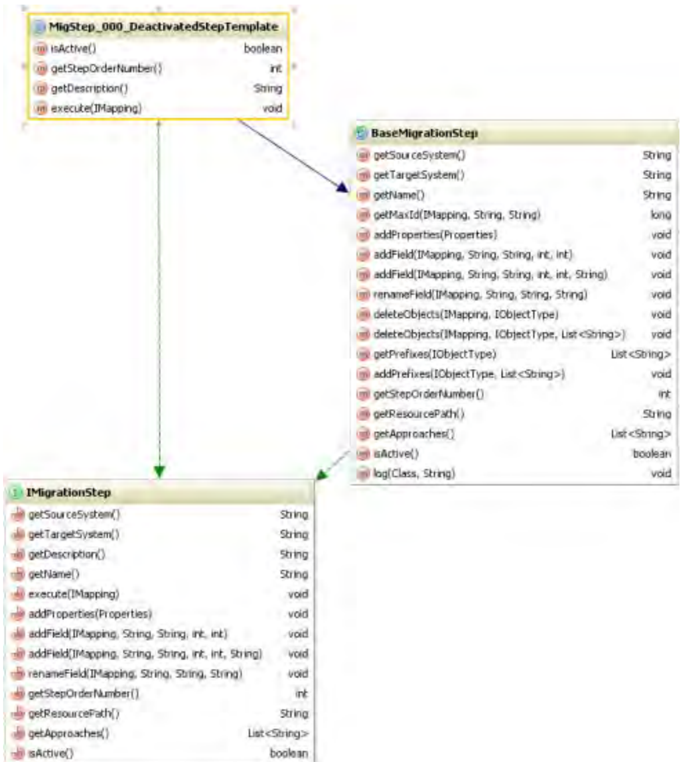
Abbildung 2: Migration-Interface
