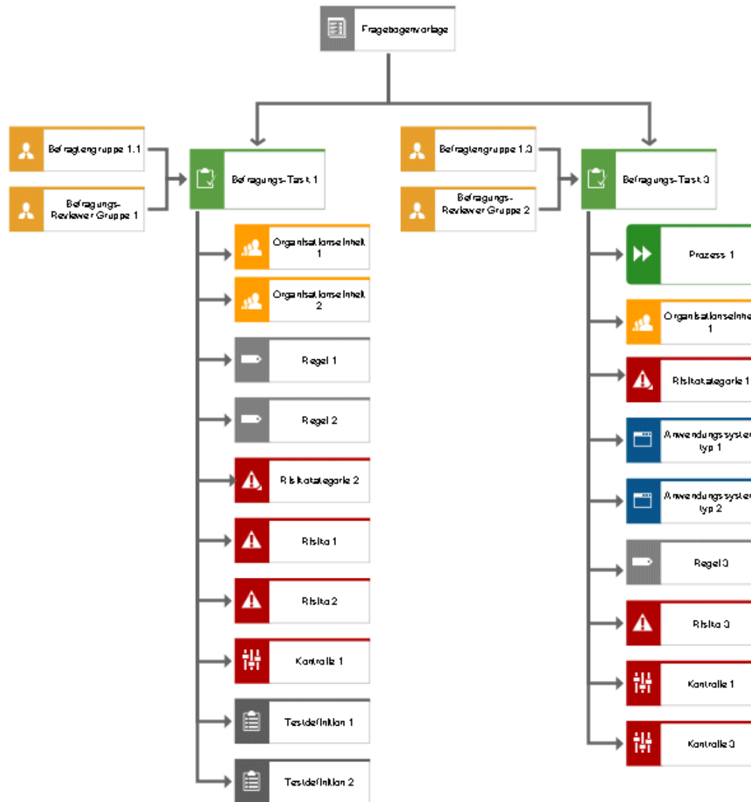
Abbildung 4: Beispiel Fragebogenvorlagenzuordnungsmodell
