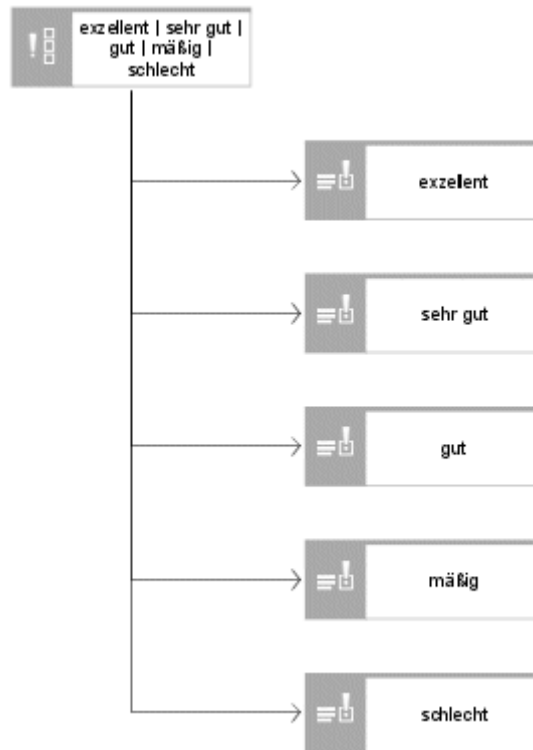
Abbildung 3: Antwort-Set (Maskendiagramm)
