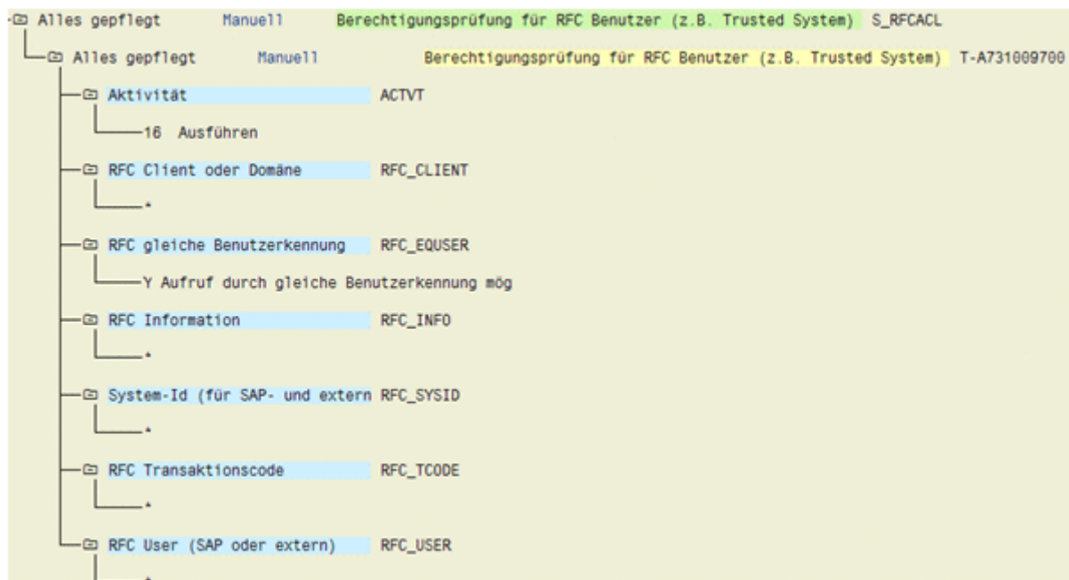
Abbildung 9: Berechtigungsobjekt 'S_RFCACL'
