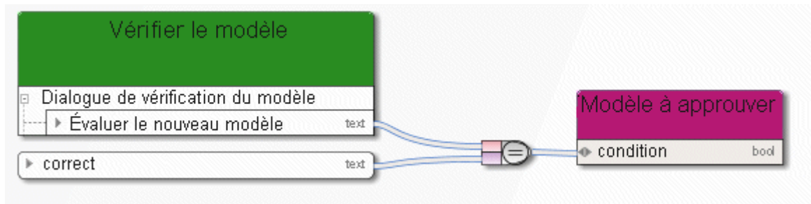
Figure 90: Égal à
