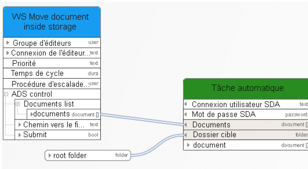
Figure 52: Déplacer documents
