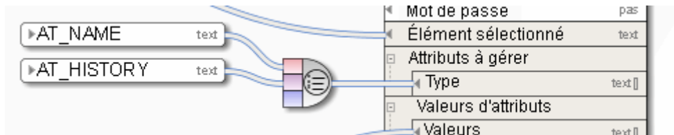
Figure 101: Créer compilation
