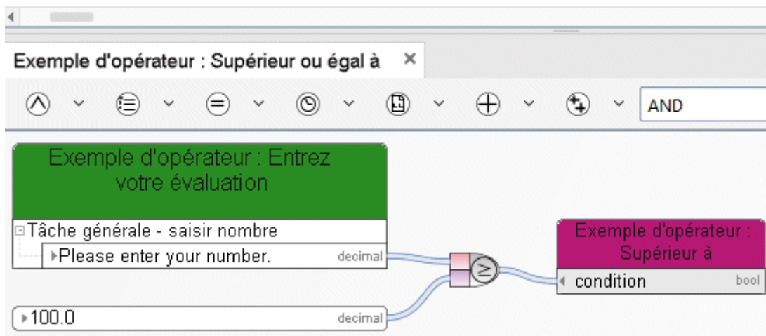
Figure 92: Supérieur à
