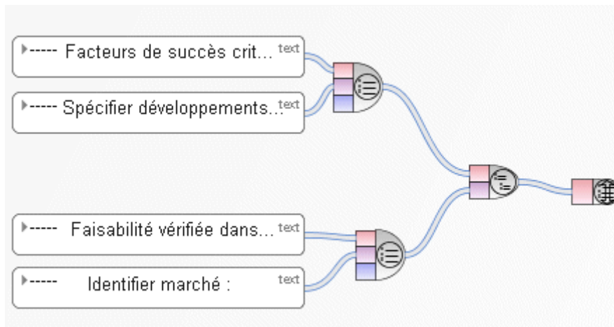
Figure 106: Fusionner compilations
