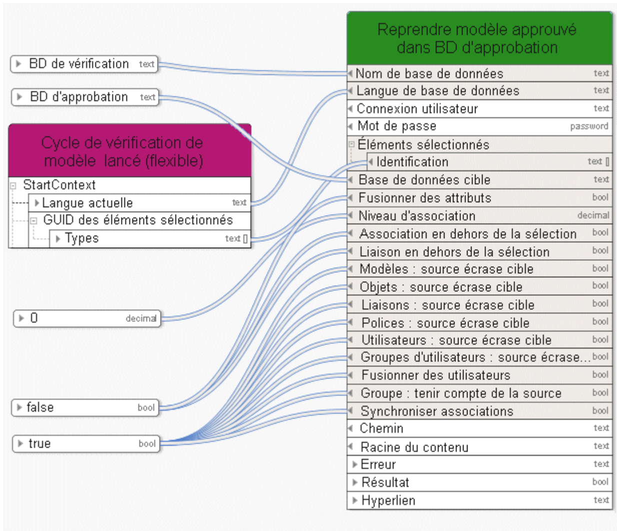
Figure 10: Fusionner modèles/objets/groupes
