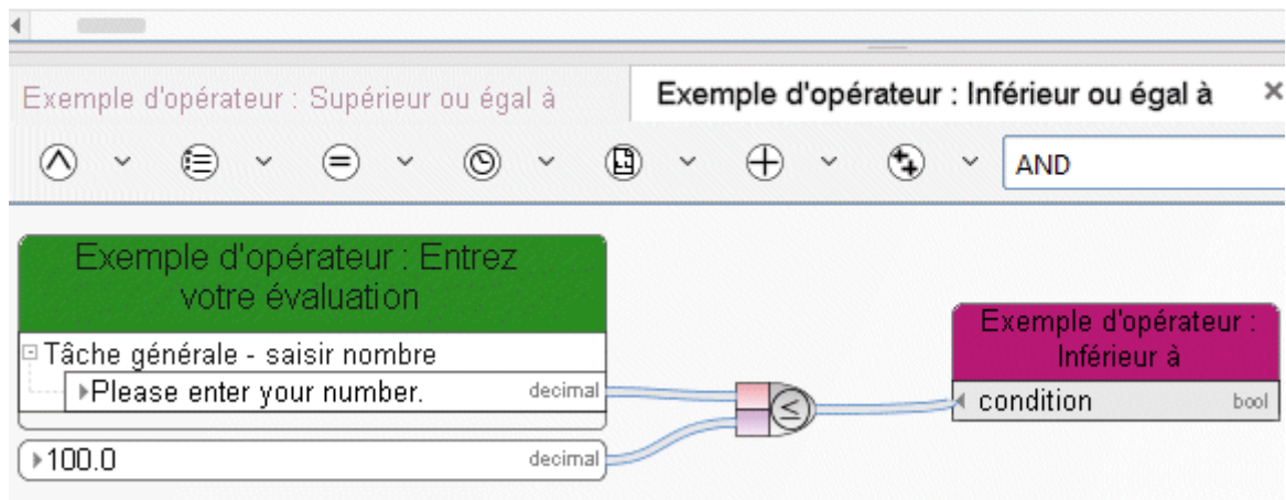
Figure 94: Inférieur à
