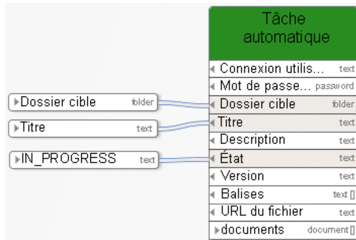
Figure 47: Créer document
