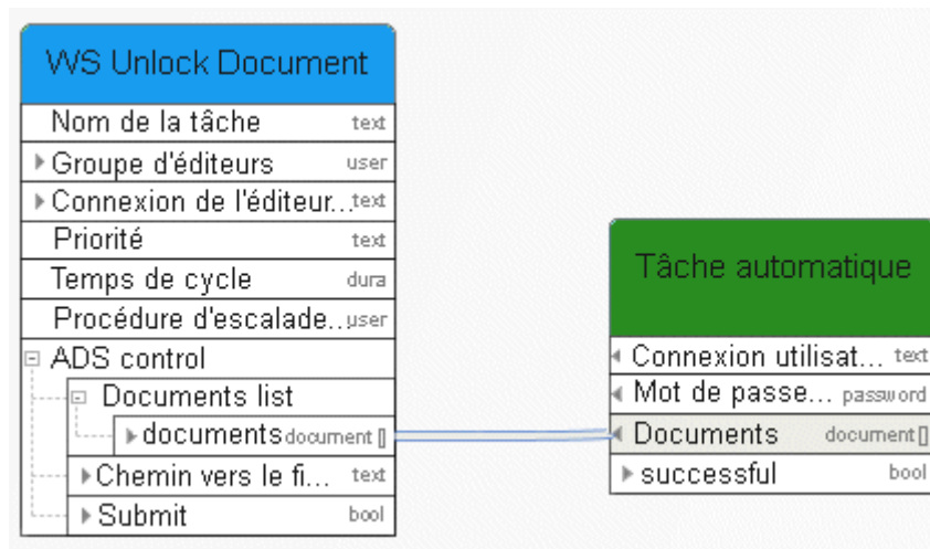
Figure 55: Déverrouiller documents
