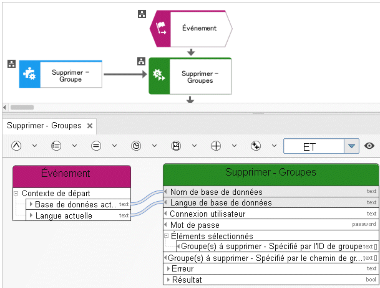
Figure 25: Supprimer groupe
