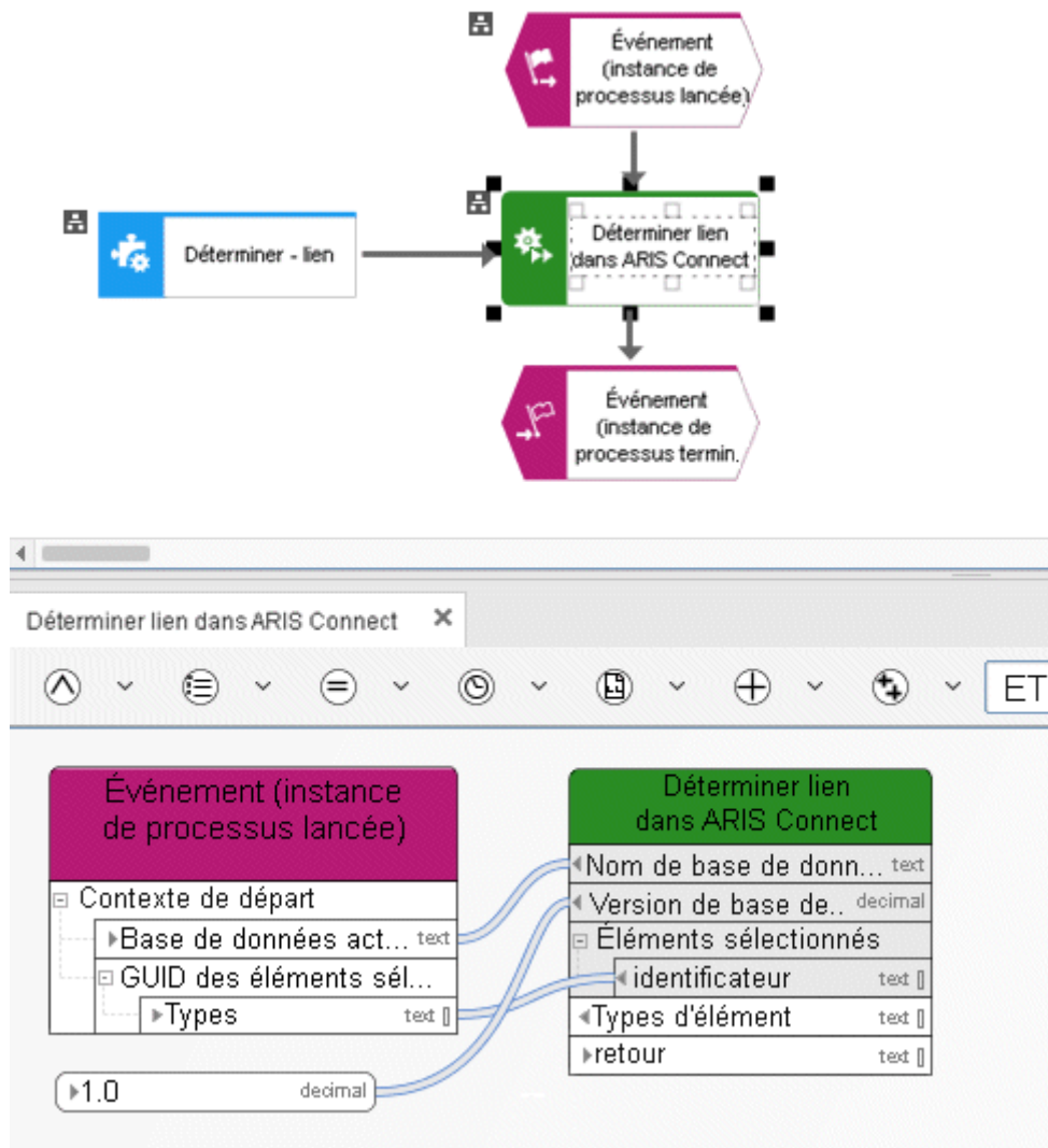
Figure 46: Déterminer - Lien
