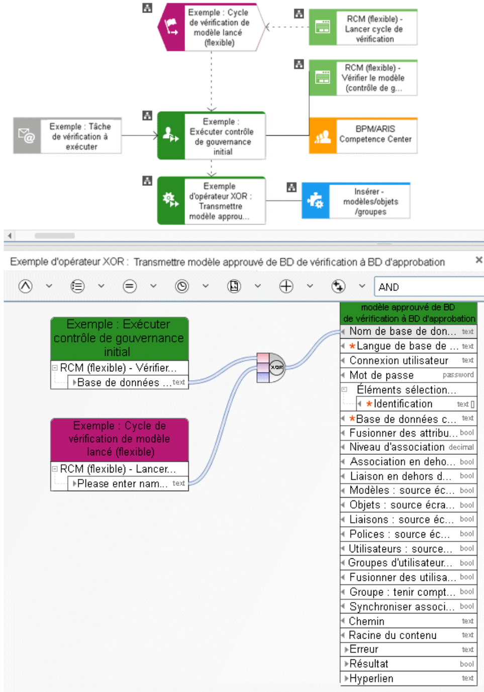
Figure 119: XOR
