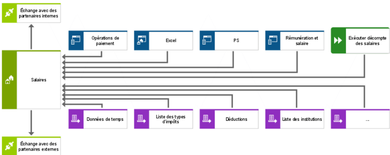
Figure 197: Liaison « assiste » entre les éléments du SI et la fonction
