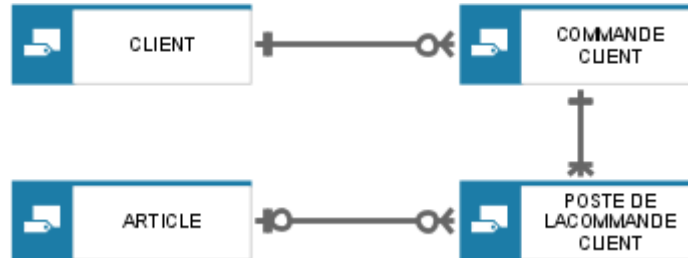
Figure 49: Modèle de données en notation IE
