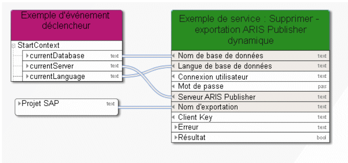
Figure 23: Supprimer une exportation ARIS Publisher dynamique
