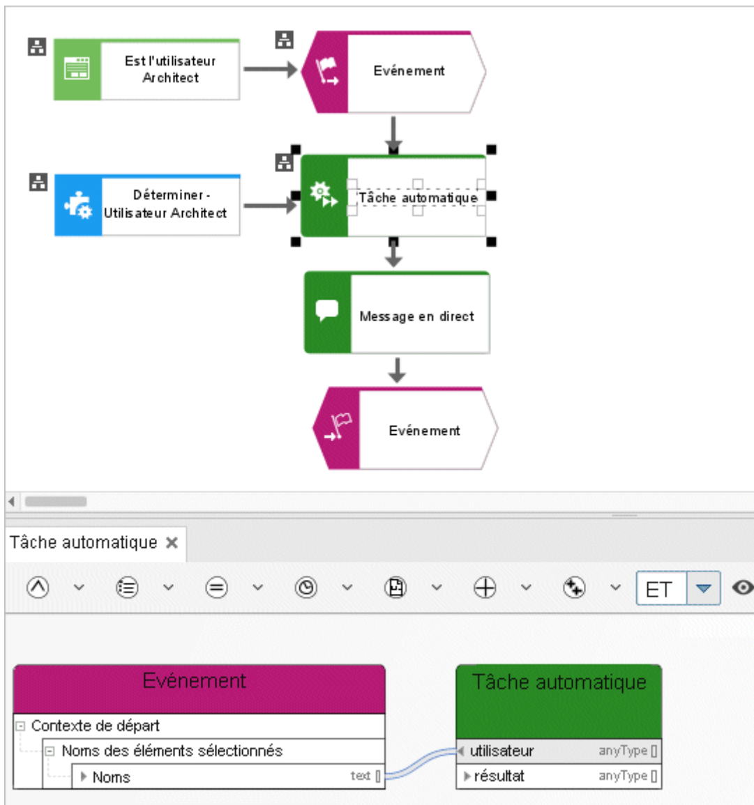
Figure 68: Extraire – utilisateur Architect
