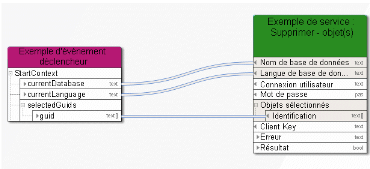
Figure 26: Supprimer des objets
