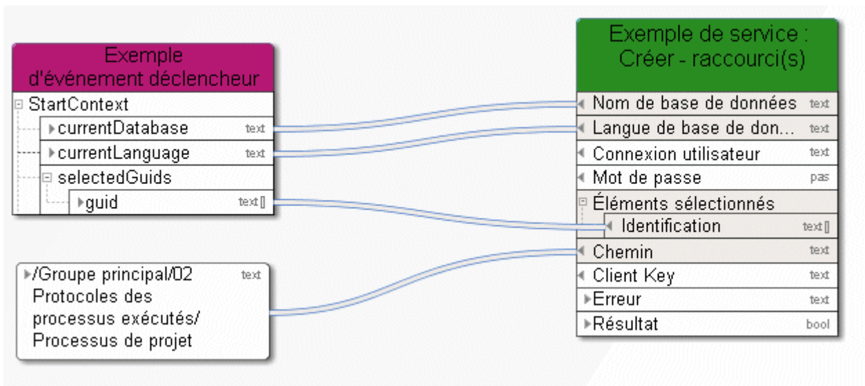
Figure 19: Créer un raccourci
