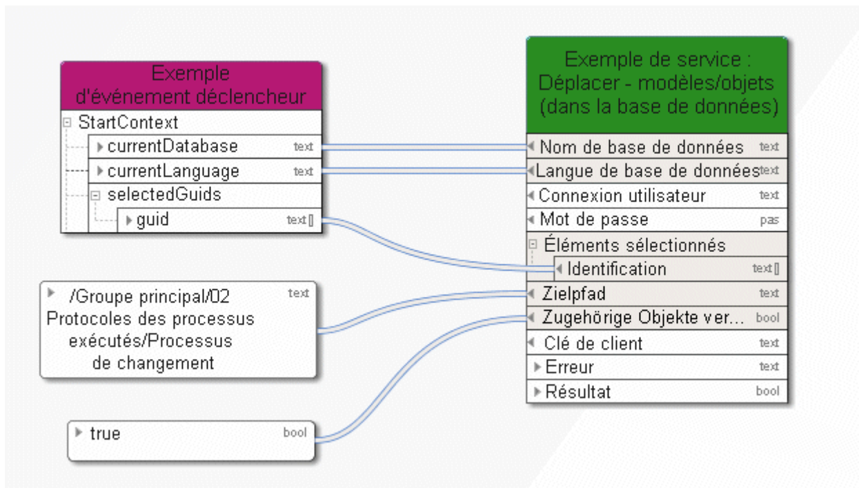
Figure 29: Déplacer des modèles/objets au sein de la base de données
