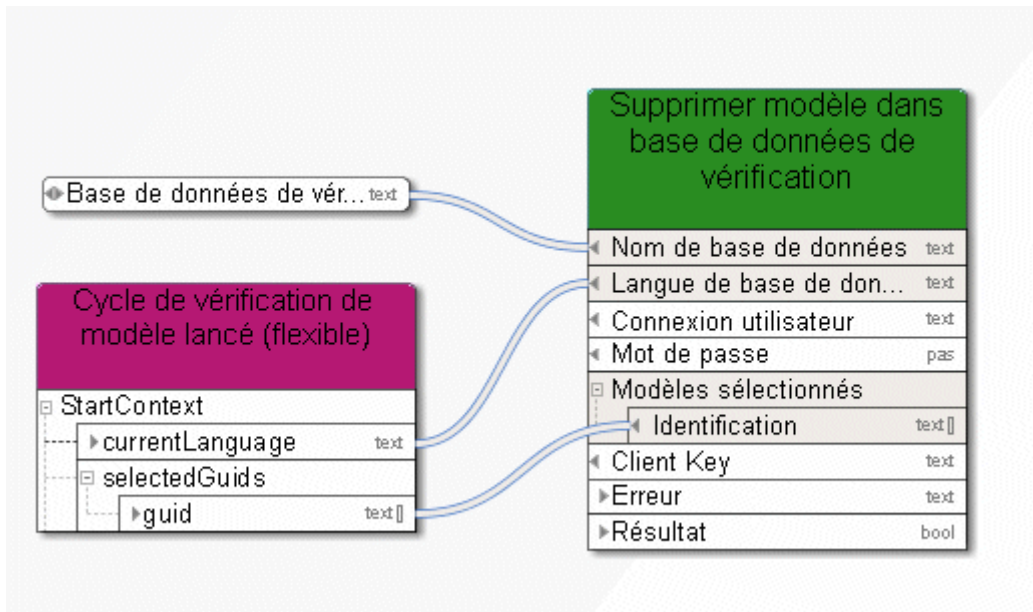
Figure 25: Supprimer les modèles
