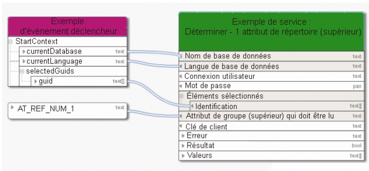
Figure 31: Lire exactement un attribut de groupe (supérieur)
