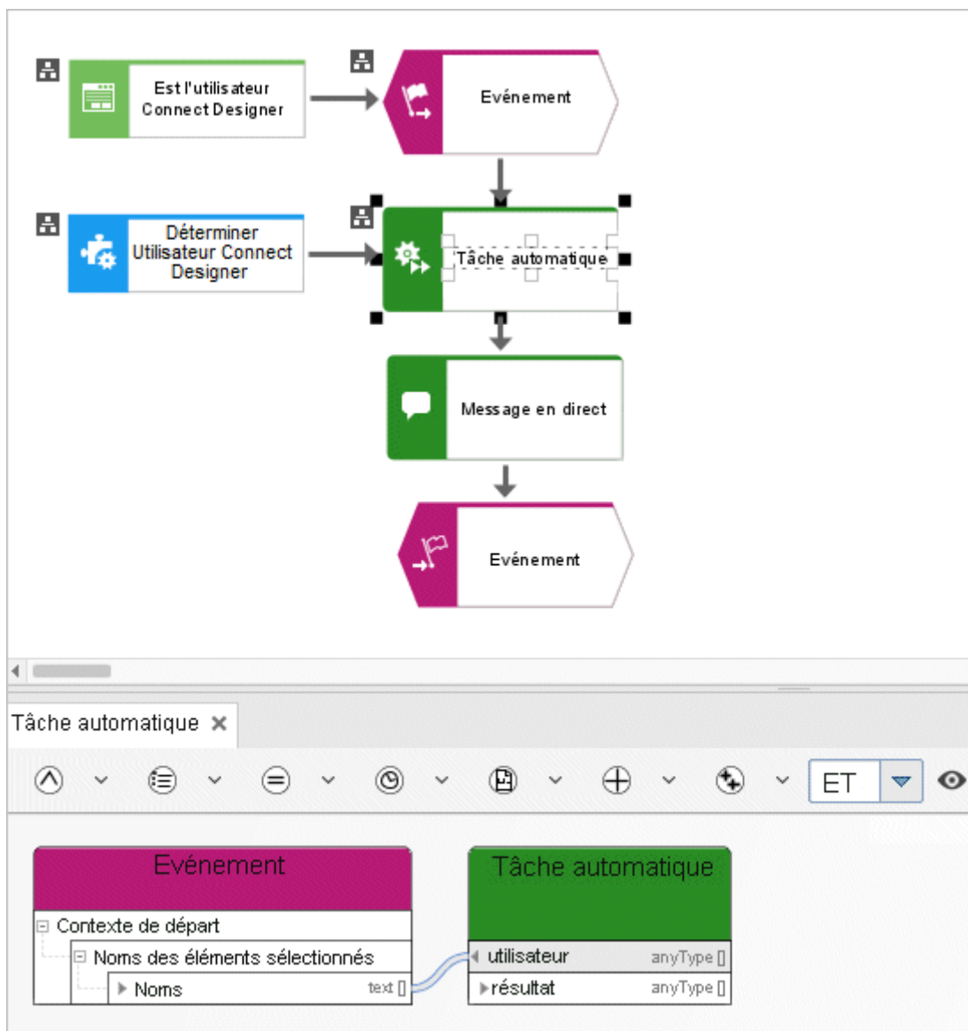
Figure 69: Extraire – utilisateur Connect Designer
