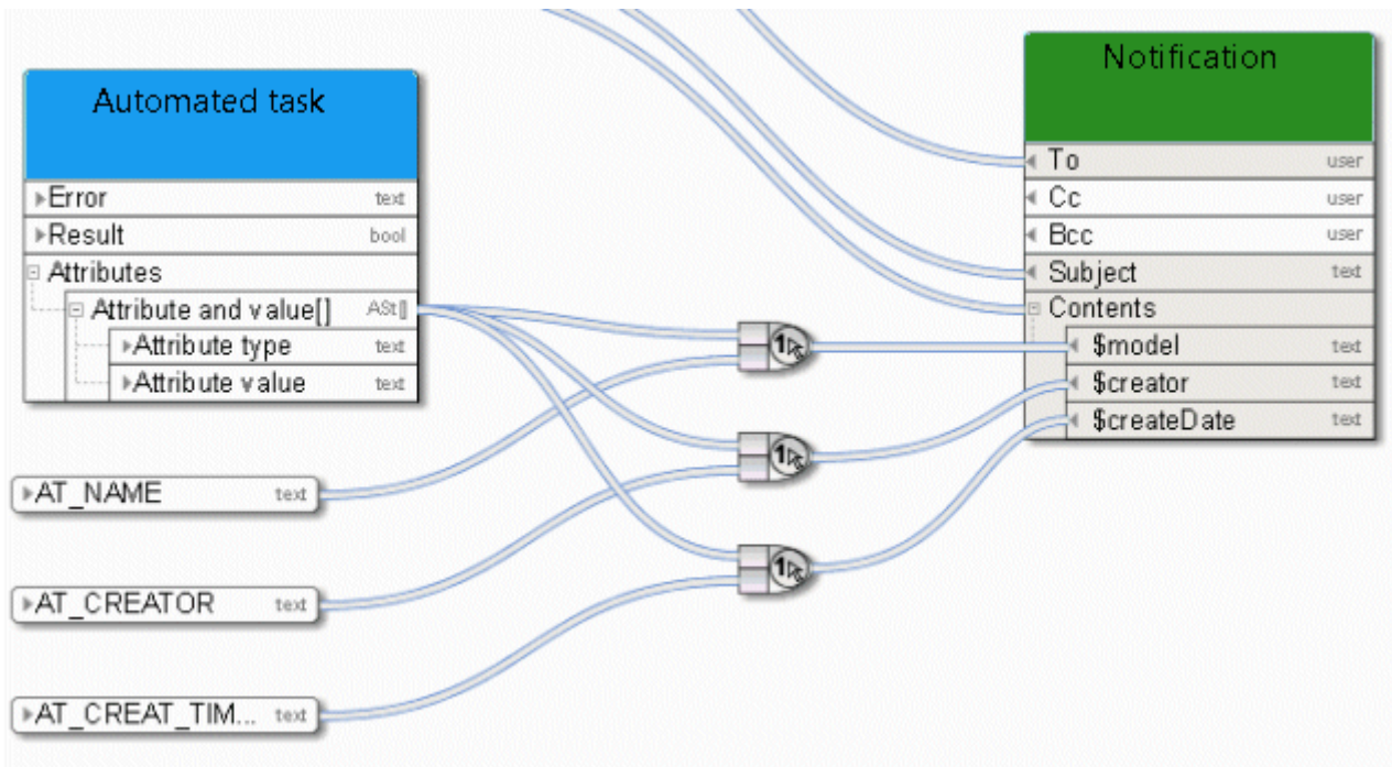
Figure 98: Sélectionner élément par ID
