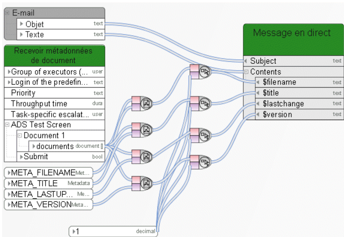
Figure 107: Recevoir métadonnées de document
