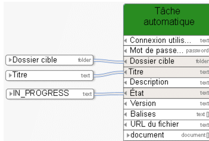
Figure 46: Créer document
