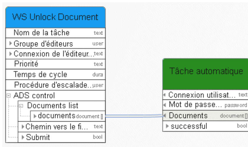
Figure 54: Déverrouiller documents
