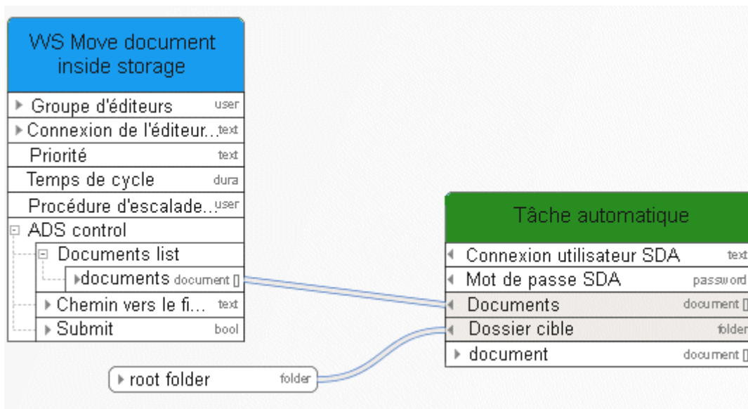
Figure 51: Déplacer documents
