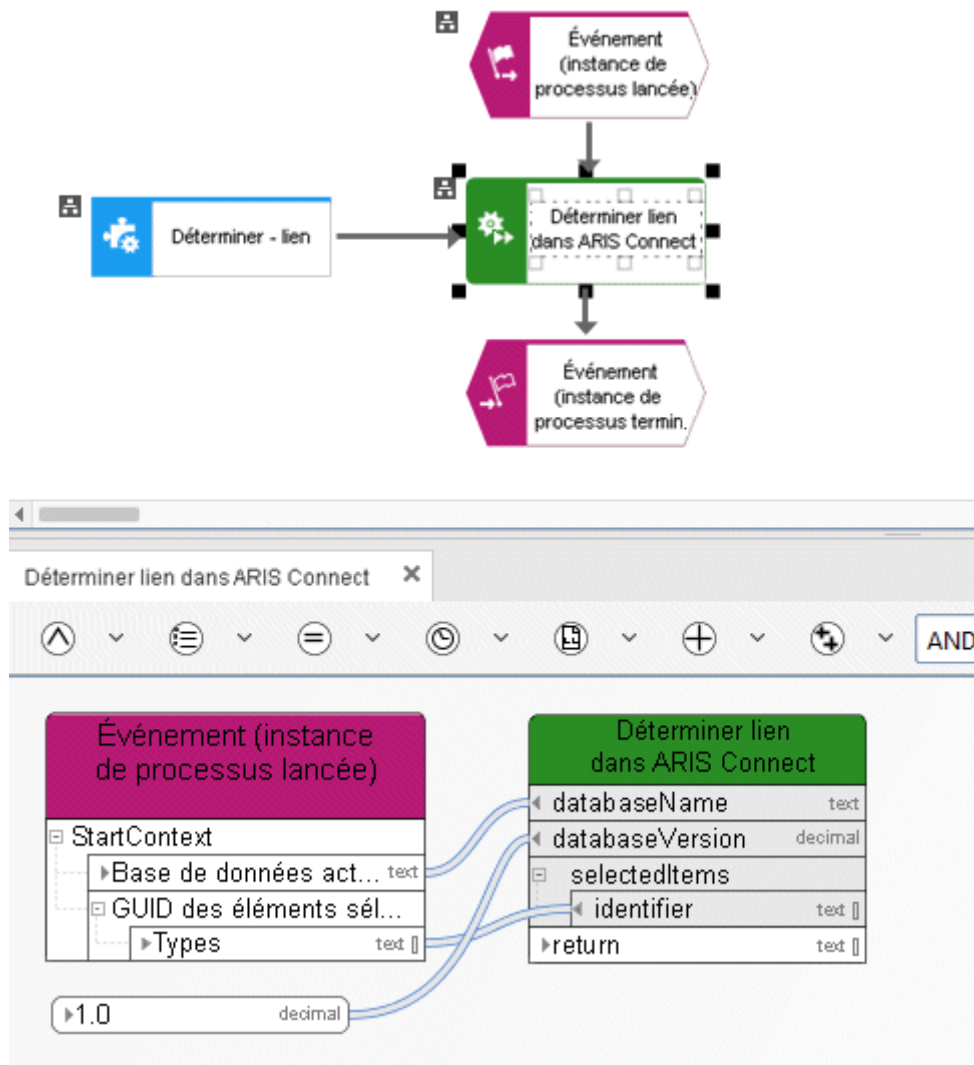
Figure 45: Déterminer - Lien
