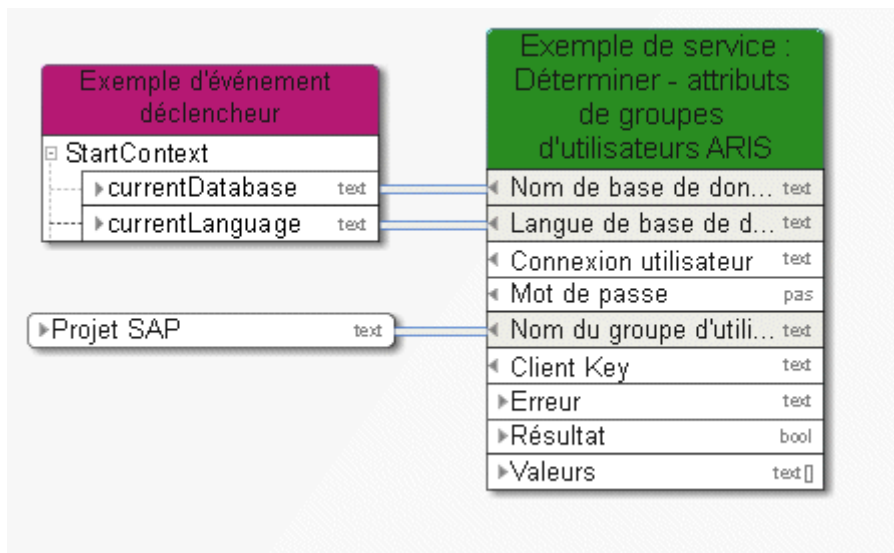
Figure 33: Déterminer les attributs du groupe d'utilisateurs ARIS
