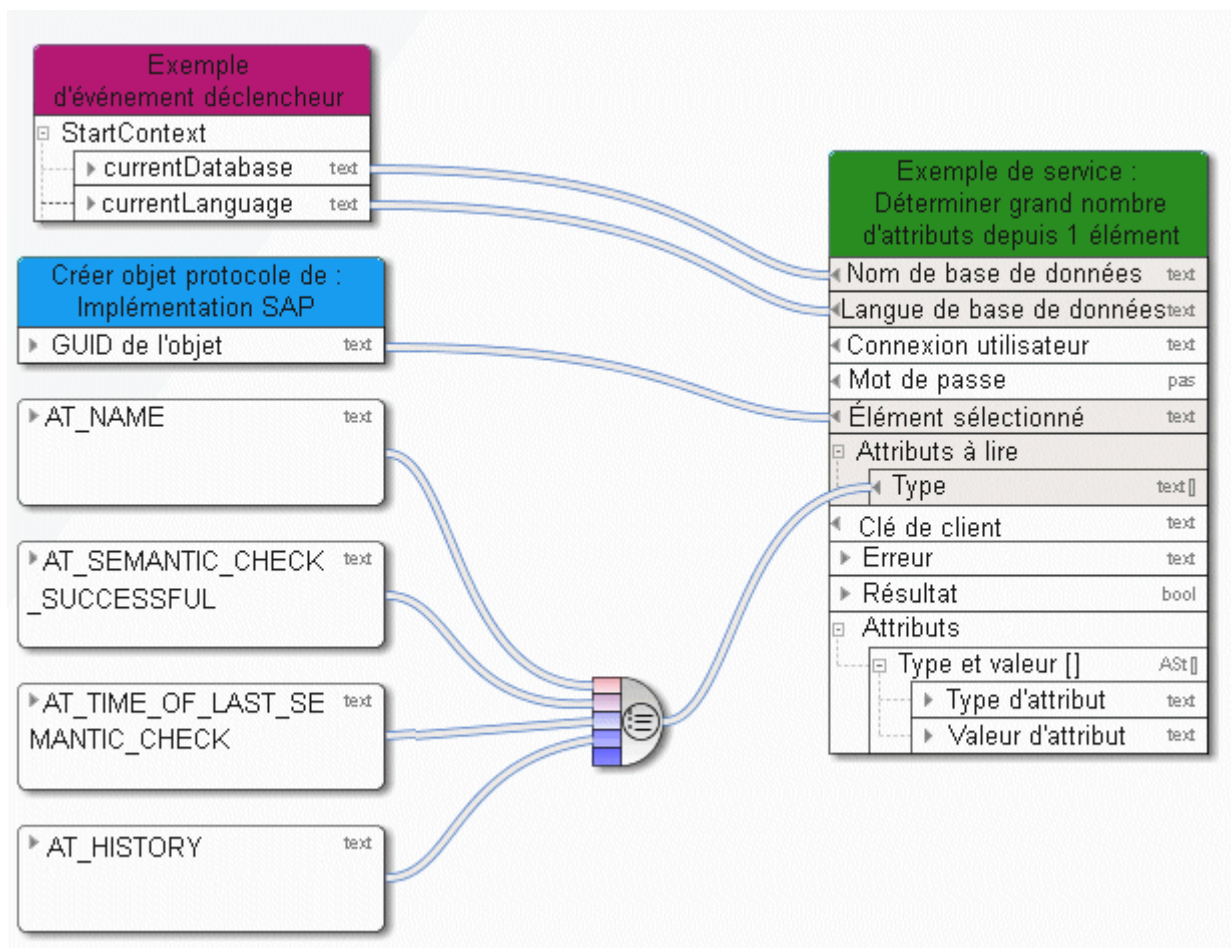
Figure 39: Déterminer plusieurs attributs d'exactly un élément
