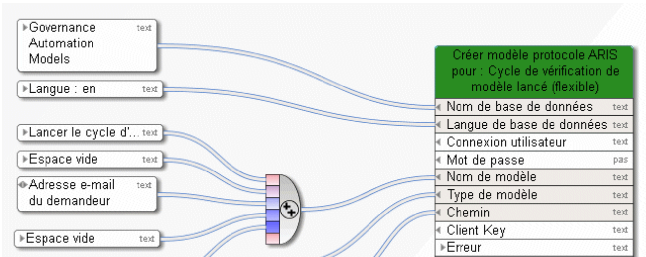
Figure 123: Exemple 1 - E-mail comme entrée
