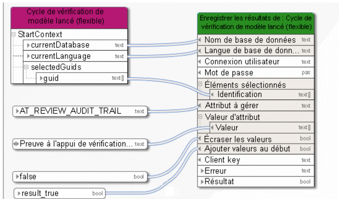
Figure 42: Gérer exactement un attribut dans plusieurs éléments
