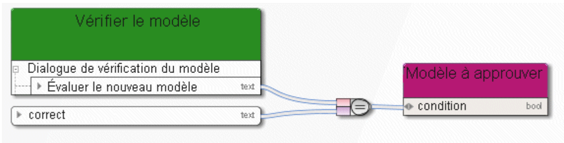
Figure 89: Égal à
