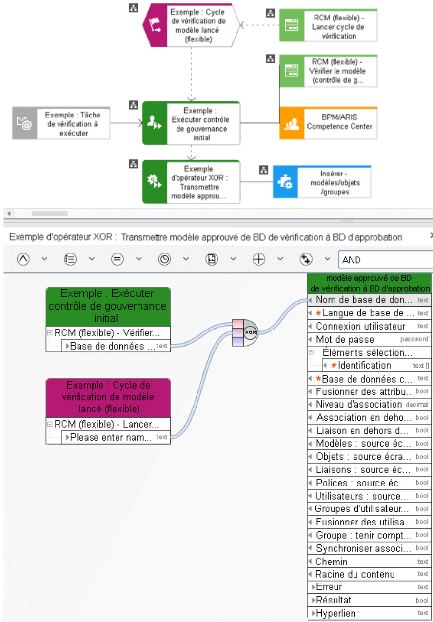
Figure 118: XOR
