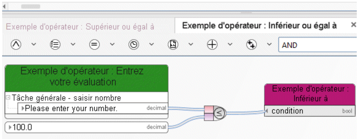
Figure 93: Inférieur à
