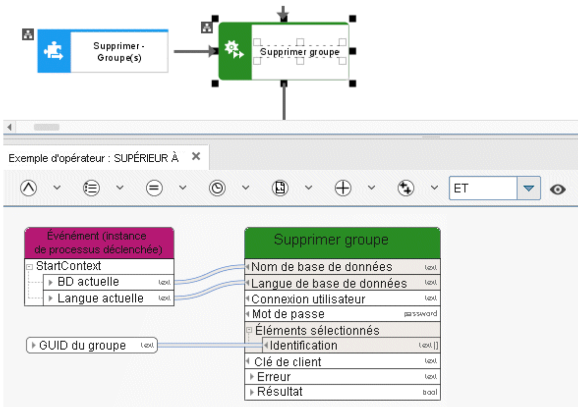
Figure 24: Supprimer groupe
