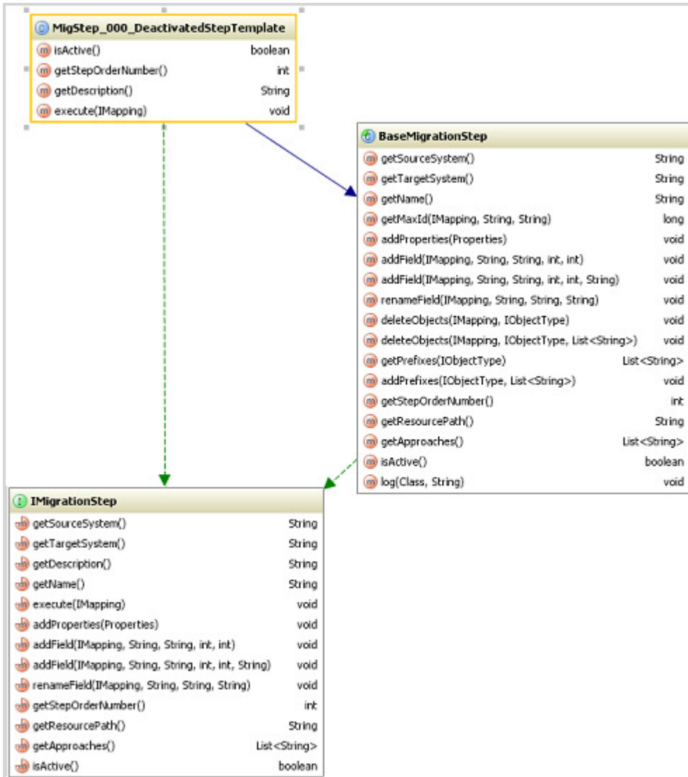
Abbildung 2: Migration-Interface
