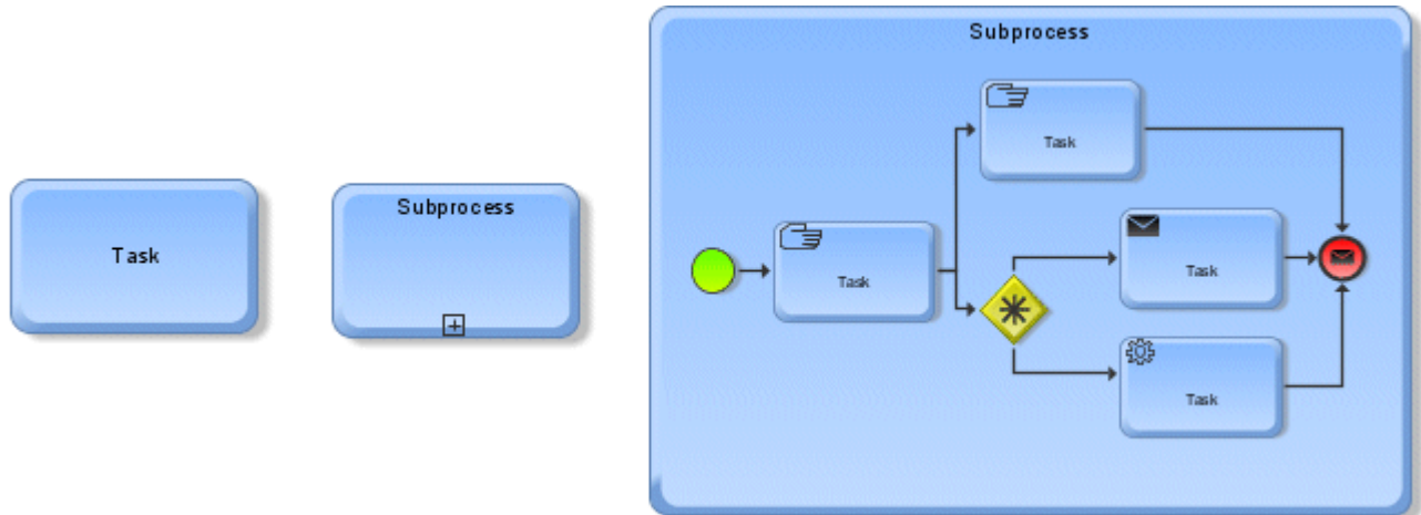
Illustration 151: Activités en langage BPMN
