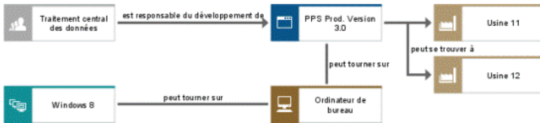
Illustration 102: Diagramme d'accès (extrait)
