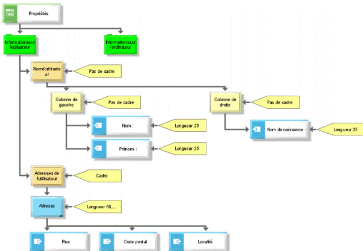
Illustration 104: Exemple d'un diagramme de masque
