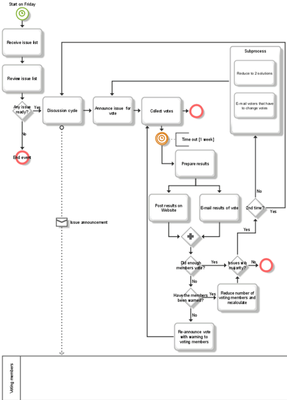
Illustration 154: Processus de vote électronique
