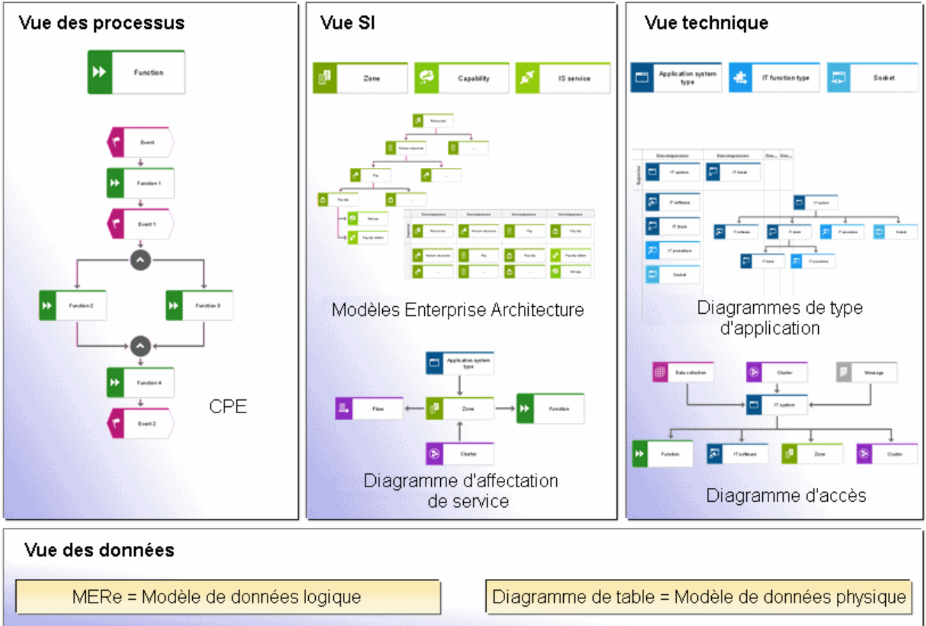
Illustration 132: Vue des processus, vue SI et vue technique
