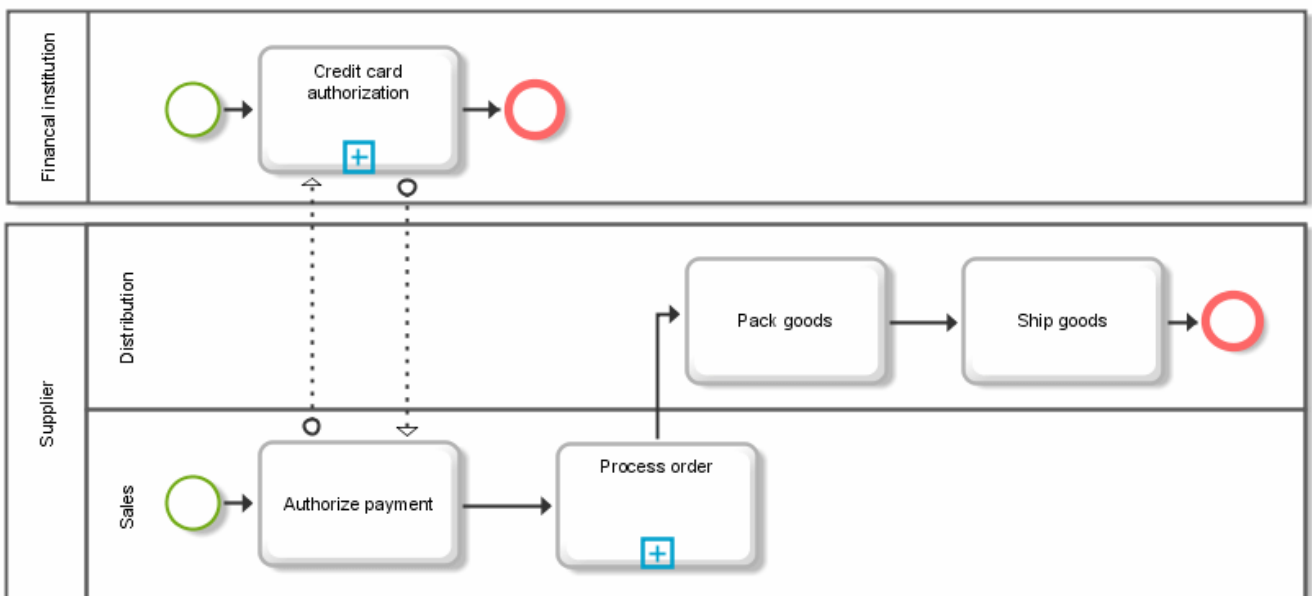
Illustration 144: Deux partitions avec un flux de séquence et un flux de message
