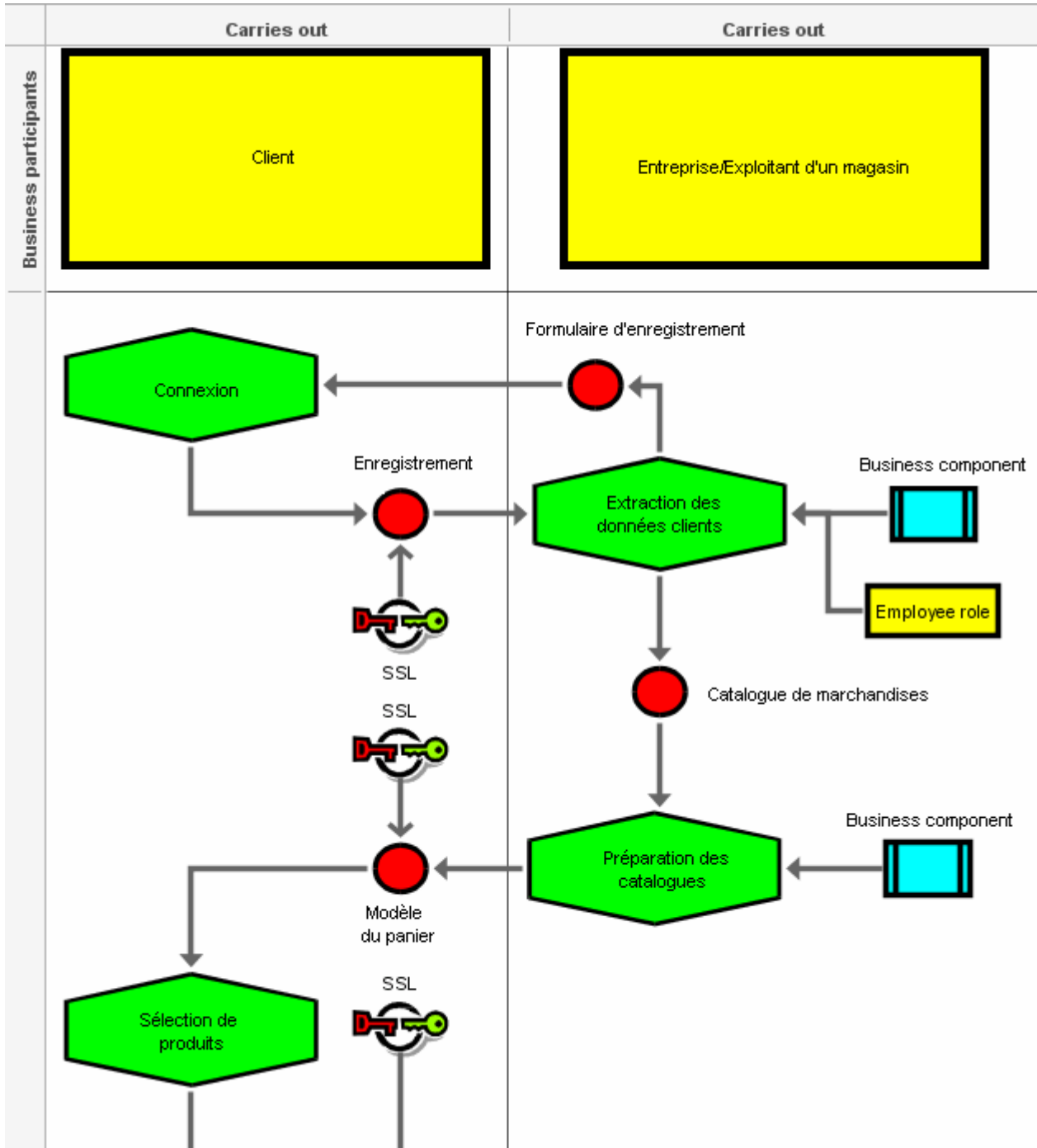
Illustration 130: Extrait du e-Business scenario "Magasin en ligne"
