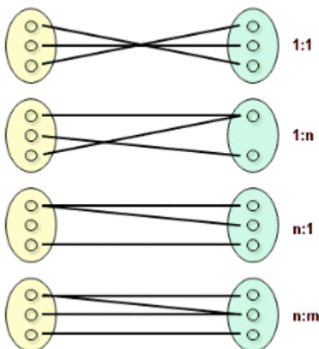
Illustration 25: Cardinalités des relations entre deux types d'entités
