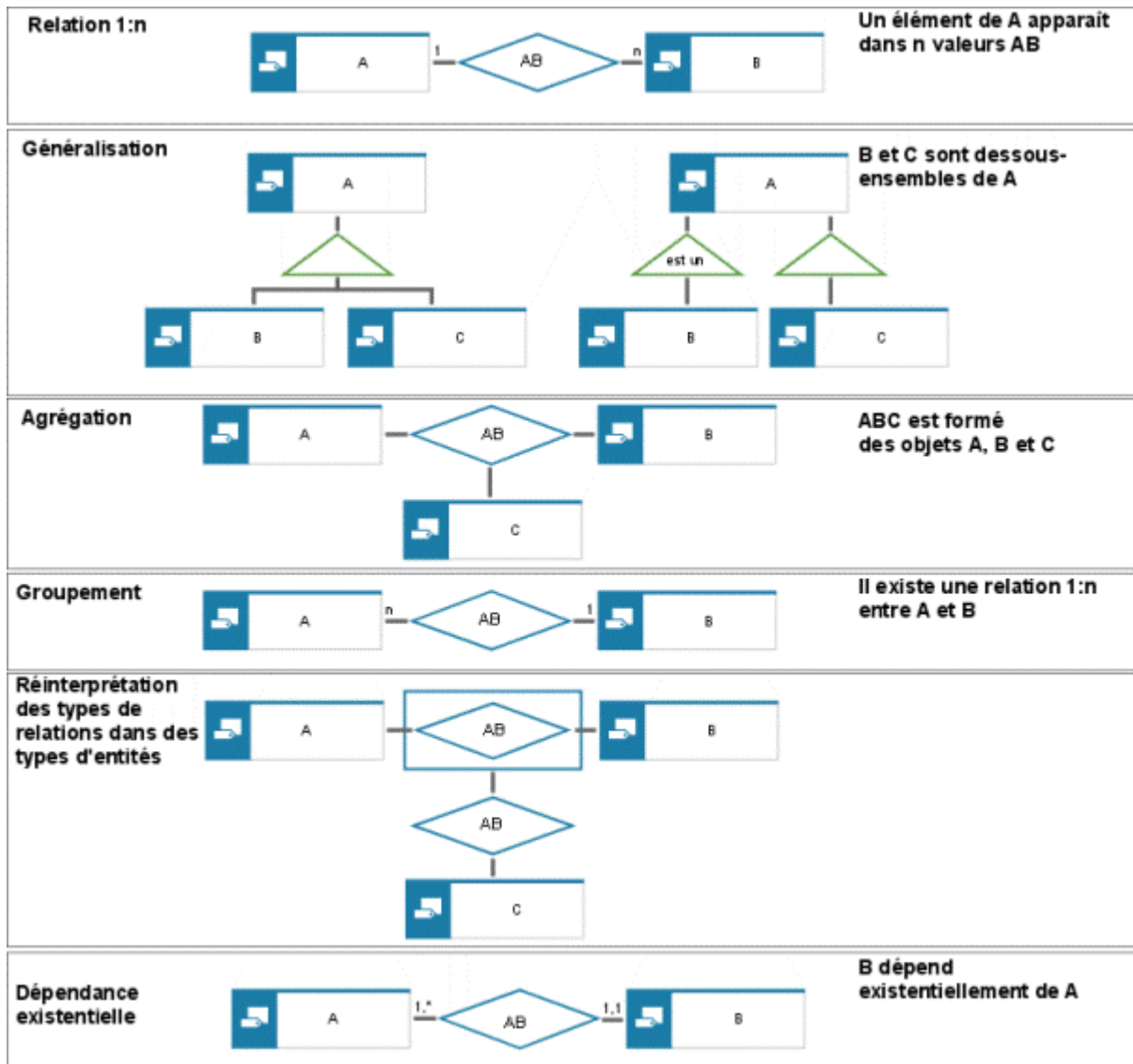
Illustration 47: Termes et formes de représentations du MERe
