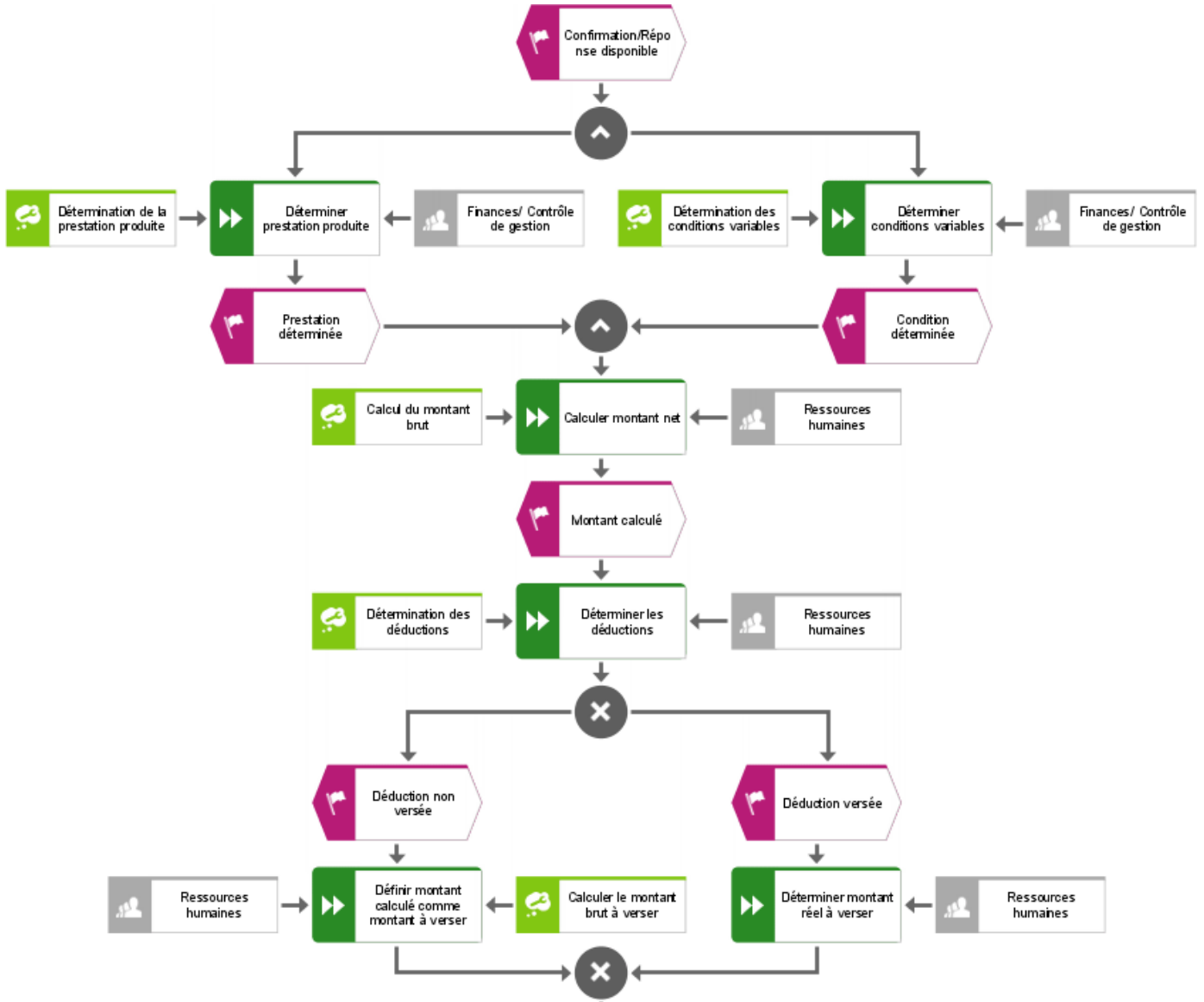
Illustration 143: Intégration des éléments SI et informatiques dans un déroulement chronologique
