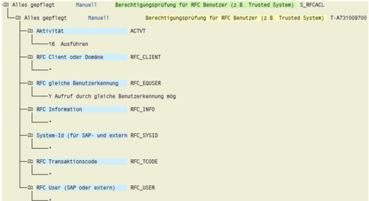
Abbildung 7: Berechtigungsobjekt 'S_RFCACL'
