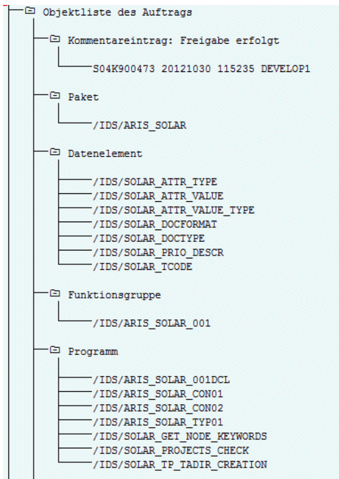
Abbildung 3: Transportauftrag: SAP®-Synchronisation (1)
