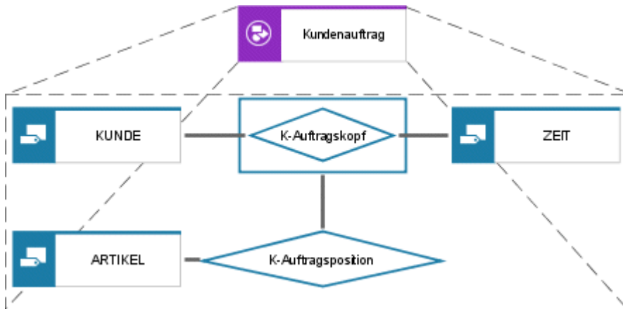
Abbildung 35: Datenclustersicht auf mehrere Objekte
