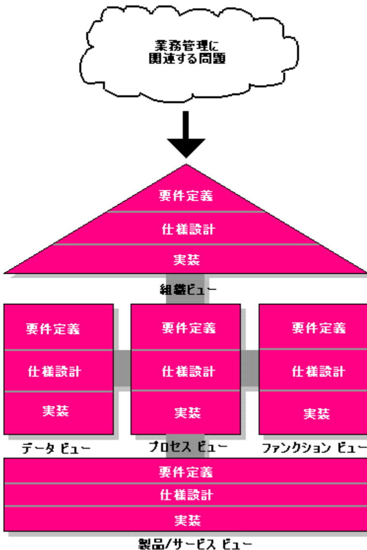
図 5: ARIS の概念
