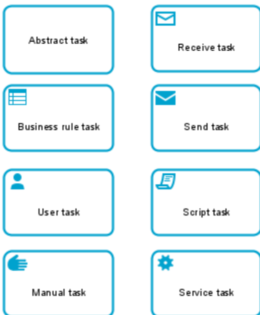
図 222: Task symbols
