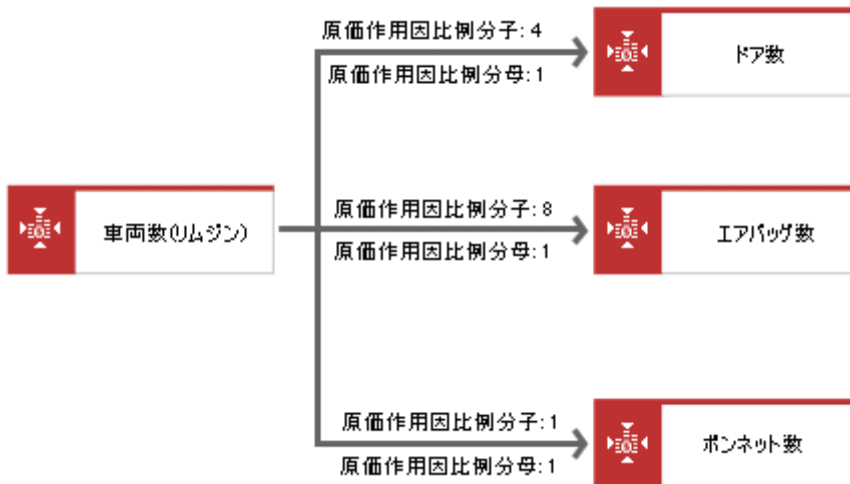
図 59: CD 図の例
