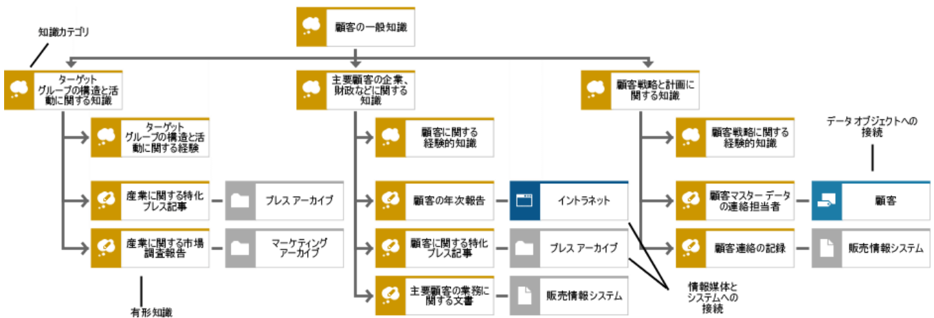
図 178: 知識構造図
