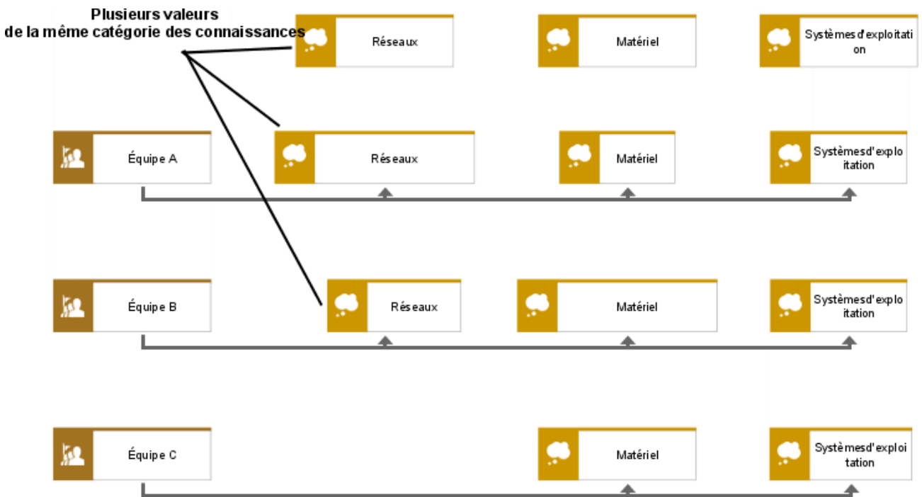
Illustration 180: Carte des connaissances - représentation matricielle
