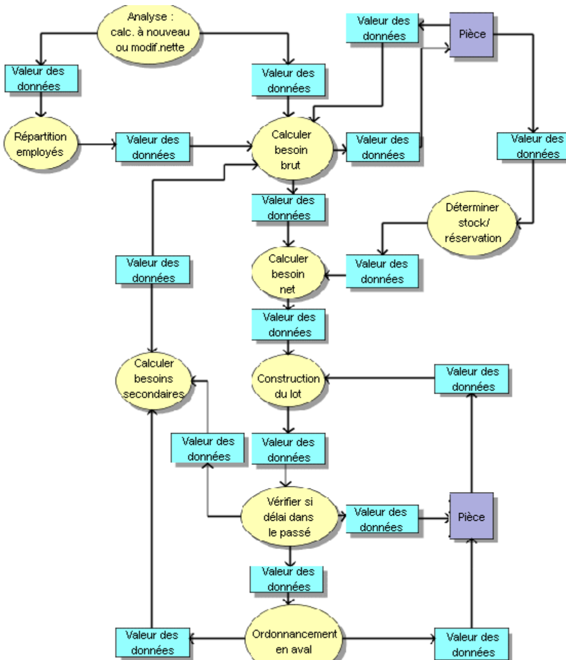
Illustration 177: Exemple de modèle fonctionnel OMT
