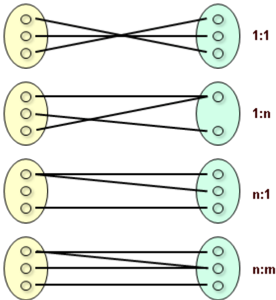
Illustration 28: Cardinalités des relations entre deux types d'entités
