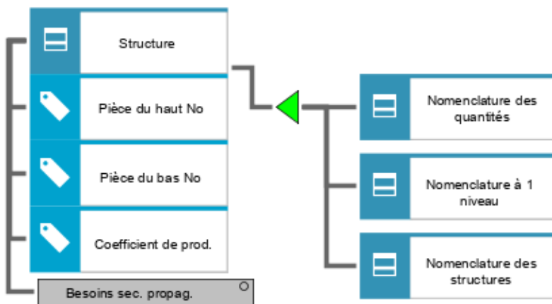
Illustration 164: Représentation de la relation généralisation/spécialisation entre classes
