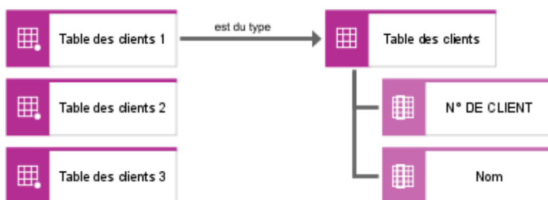
Illustration 72: Exemplaire de table
