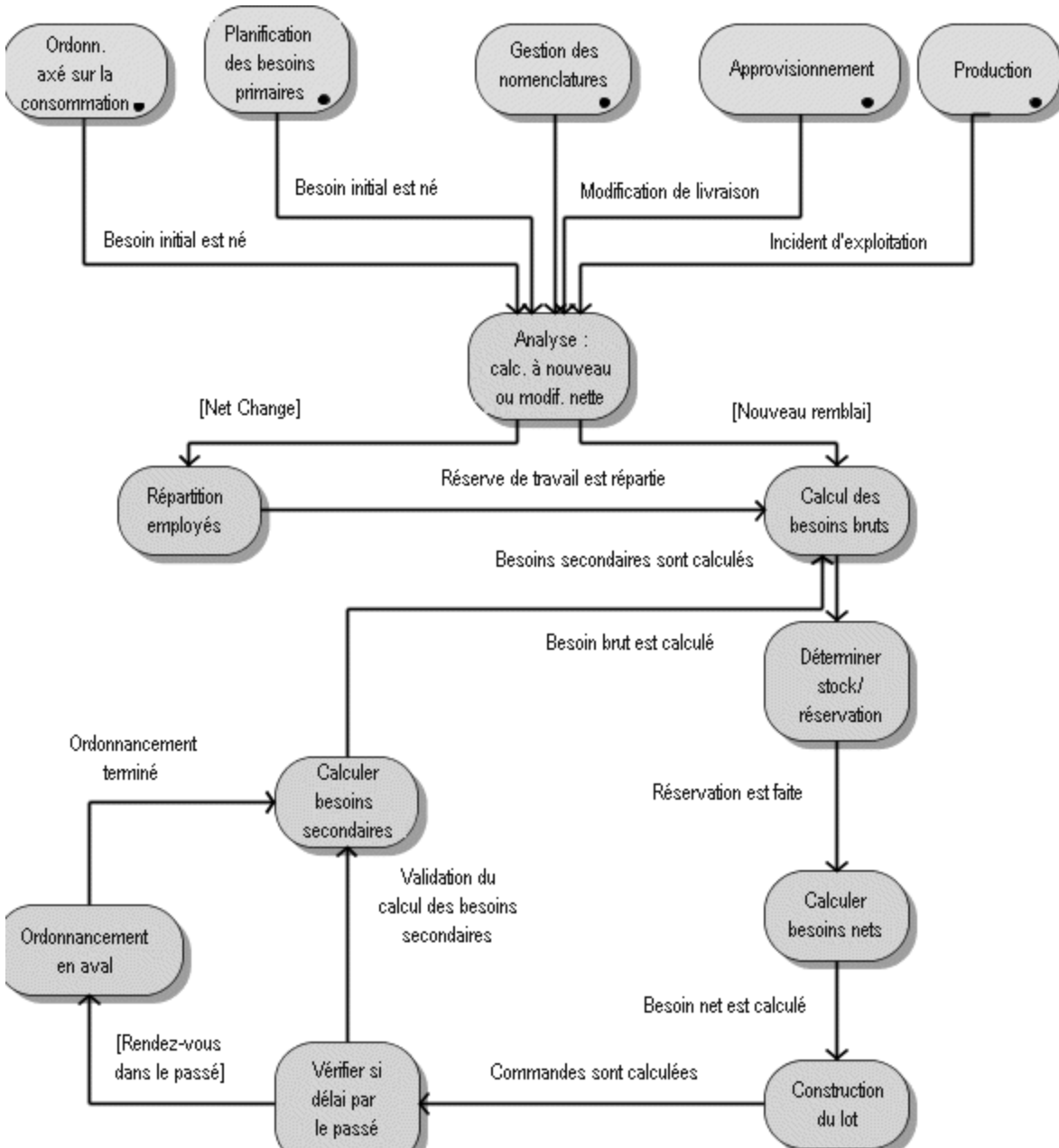
Illustration 171: Exemple de modèle dynamique OMT
