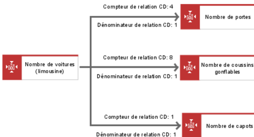
Illustration 59: Exemple d'un diagramme CD
