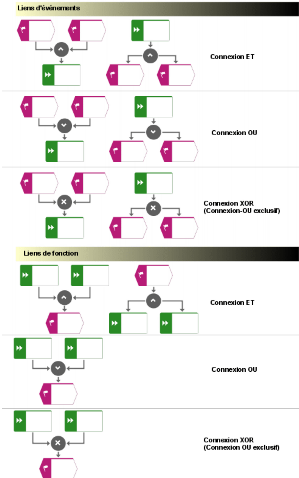
Illustration 90: Opérateurs de connexion (règles)
