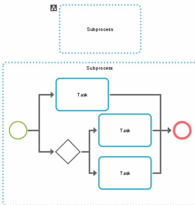
Illustration 224: Symboles d'un sous-processus d'événement
