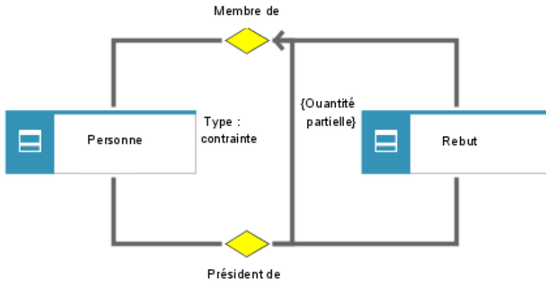
Illustration 166: Représentation des contraintes dans les associations
