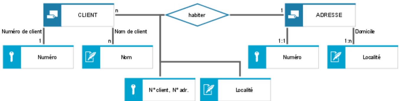
Illustration 31: Affectation d'attributs dans le MER
