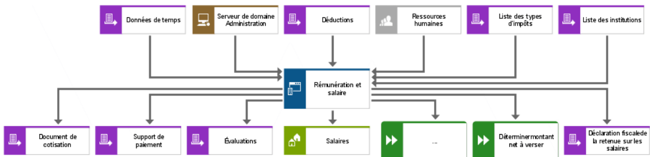
Illustration 201: Description détaillée des éléments informatiques dans le diagramme d'accès
