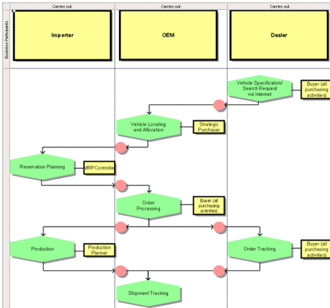
Illustration 118: Exemple d'un eBusiness scenario diagram : secteur automobile
