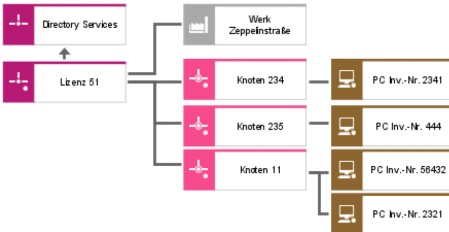
Abbildung 84: Netzdiagramm mit Hardwarekomponenten und Standortzuordnung
