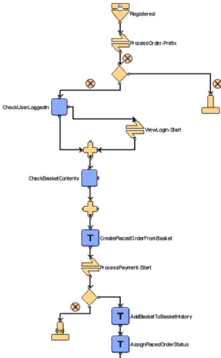
Abbildung 190: Ausschnitt aus dem Pipeline Diagram
