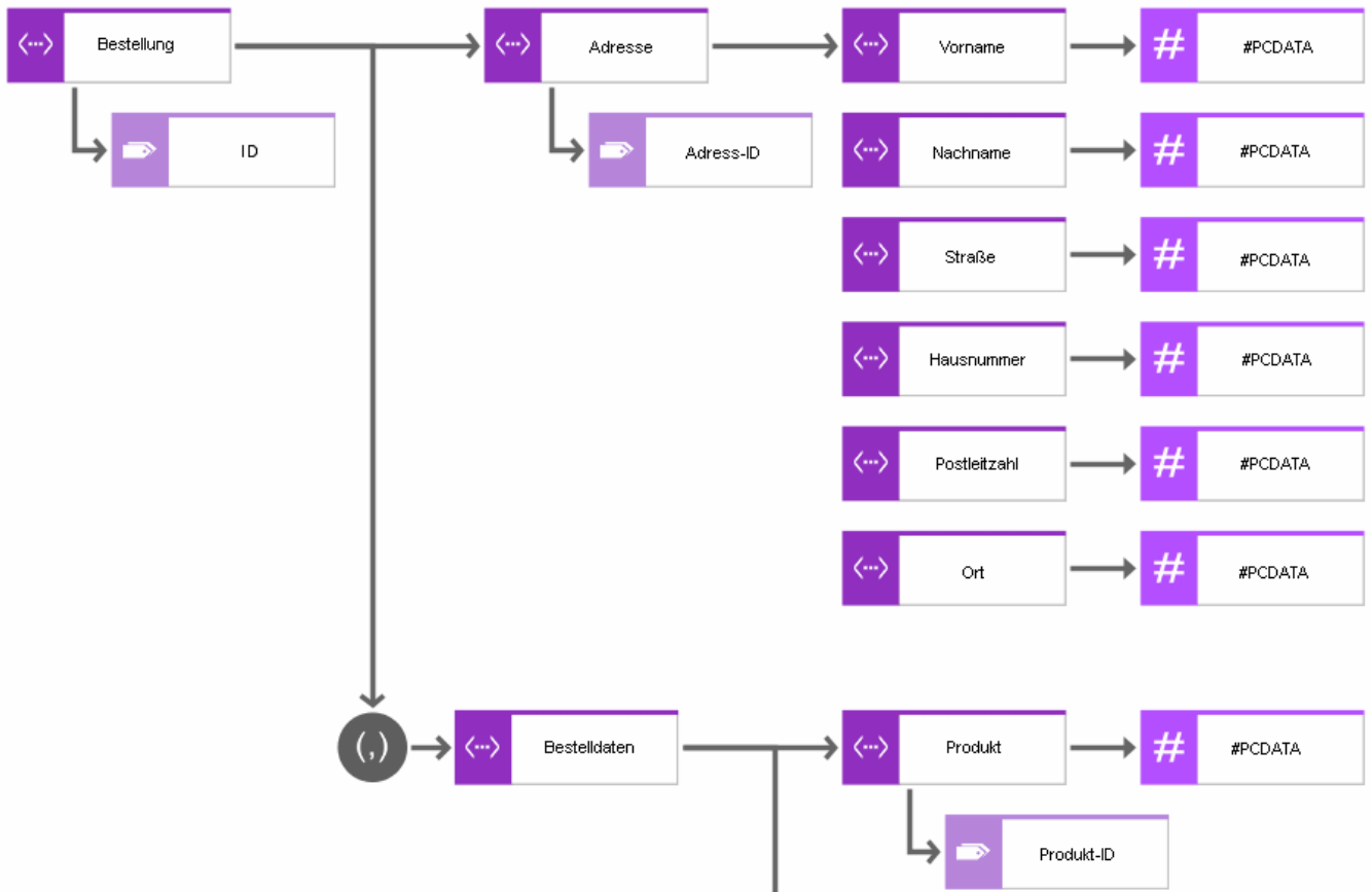
Abbildung 191: Ausschnitt aus der DTD: Bestellung
