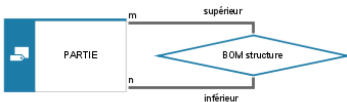
Illustration 27: MER pour une nomenclature
