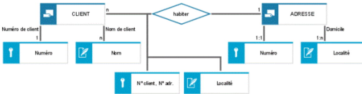
Illustration 28: Affectation d'attributs dans le MER
