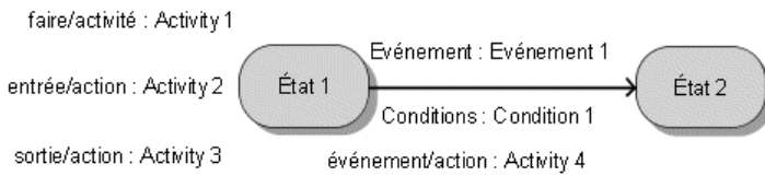
Illustration 170: Représentation d'informations complémentaires lors de la transition d'état
