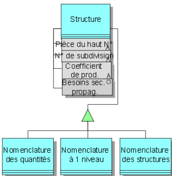
Illustration 164: Représentation de la relation généralisation/spécialisation entre classes
