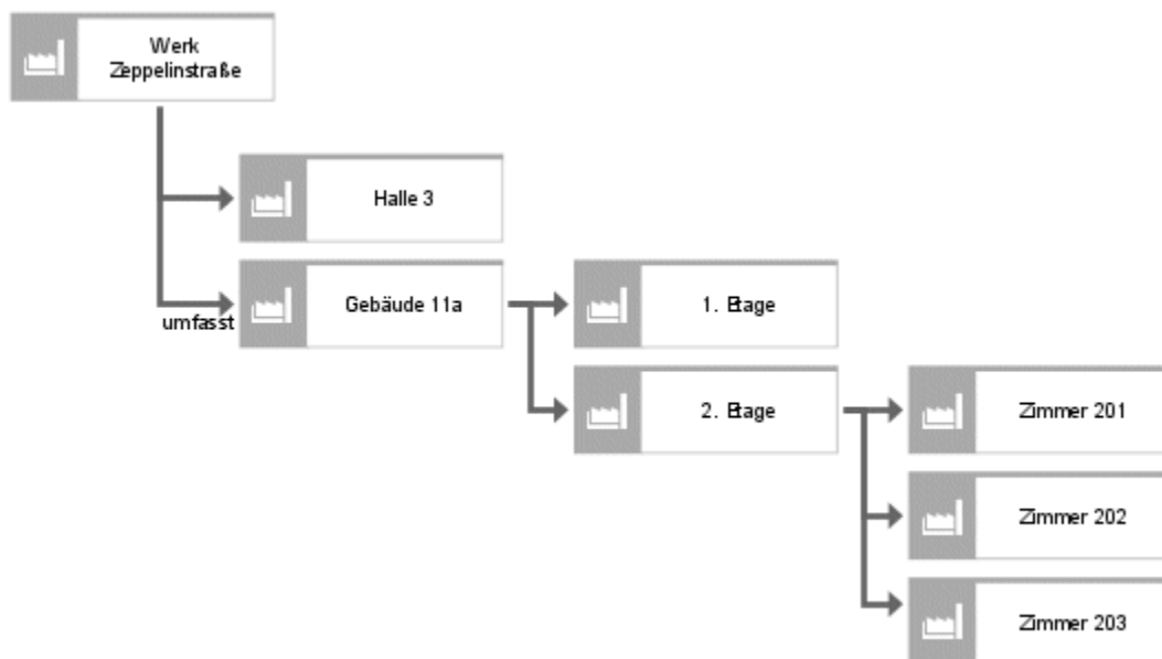
Abbildung 79: Standorthierarchien
