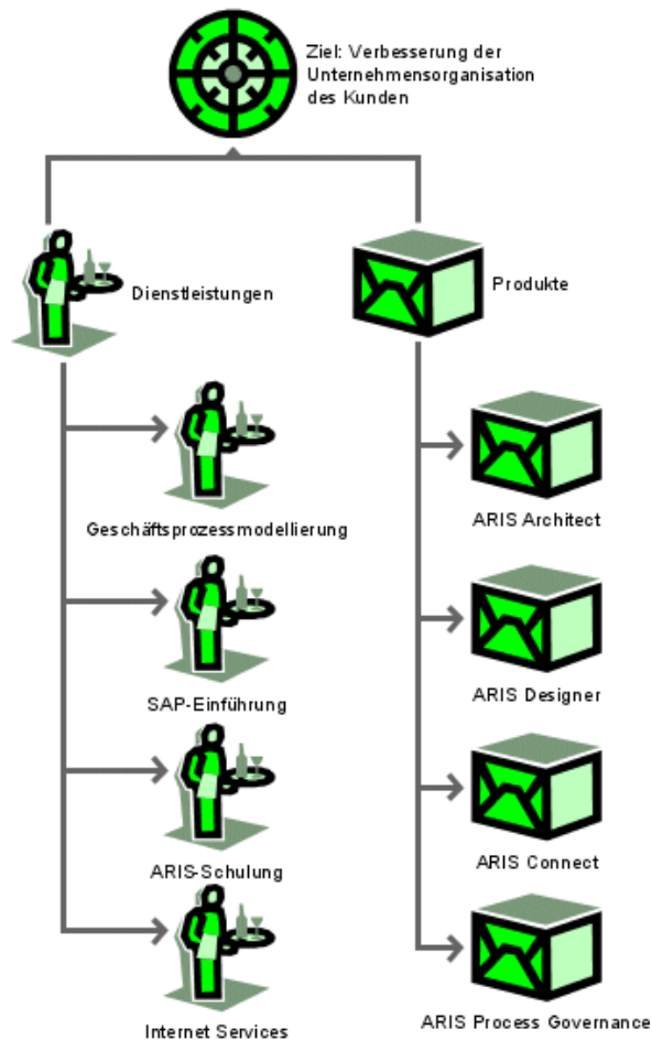
Abbildung 145: Leistungsbaum
