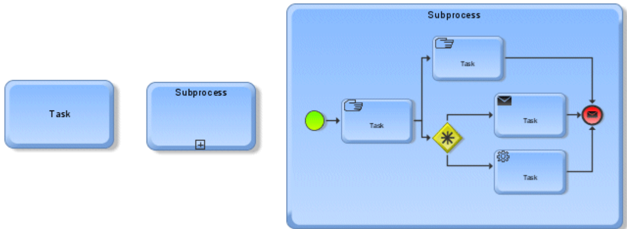
図 151: BPMN のアクティビティ
