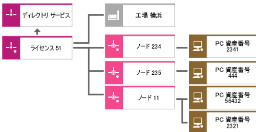
図 65: ハードウェア コンポーネントと場所の割り当てを含むネットワーク図
