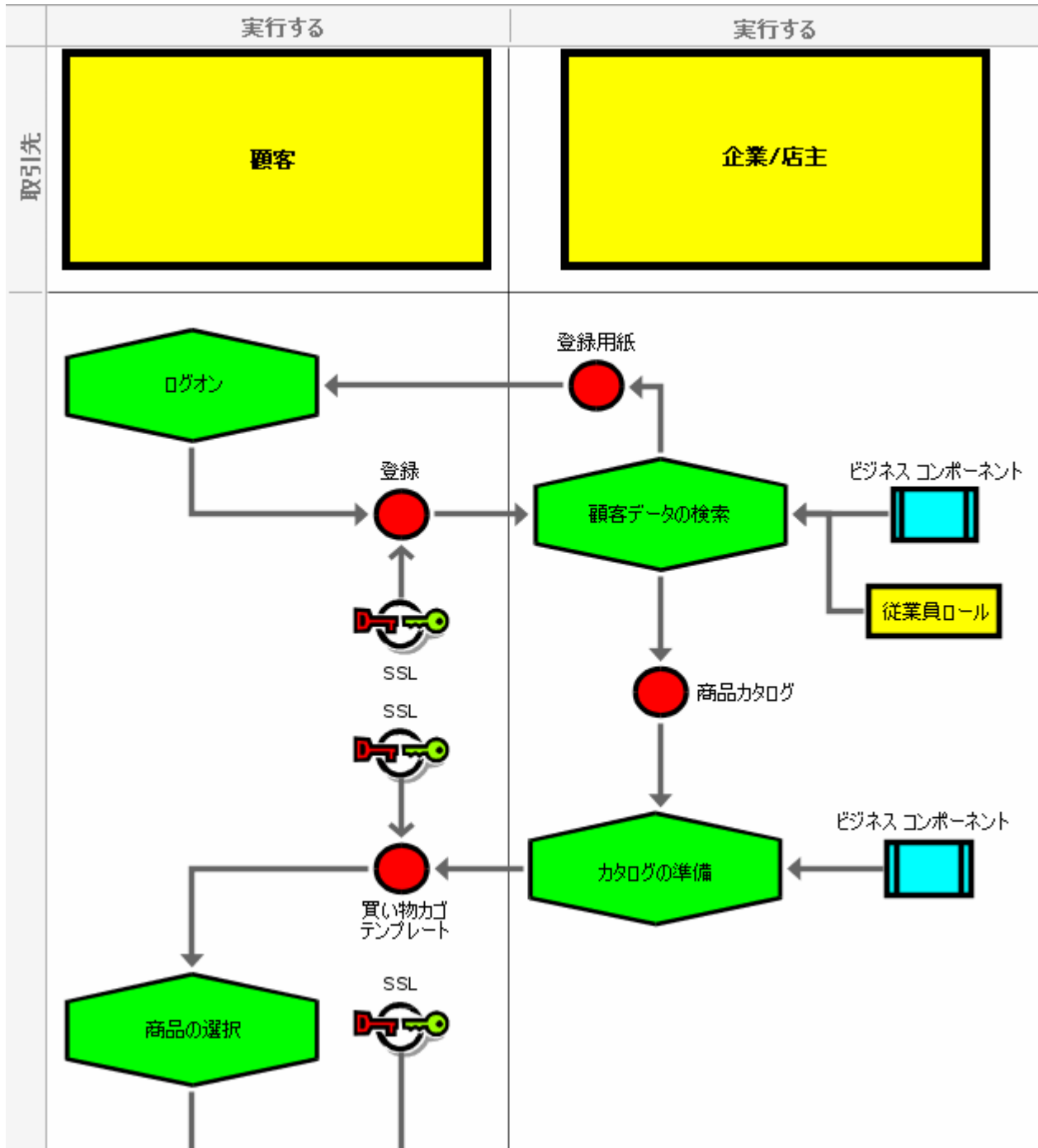
図 130: e-ビジネス シナリオ「オンライン ショップ」からの抜粋
