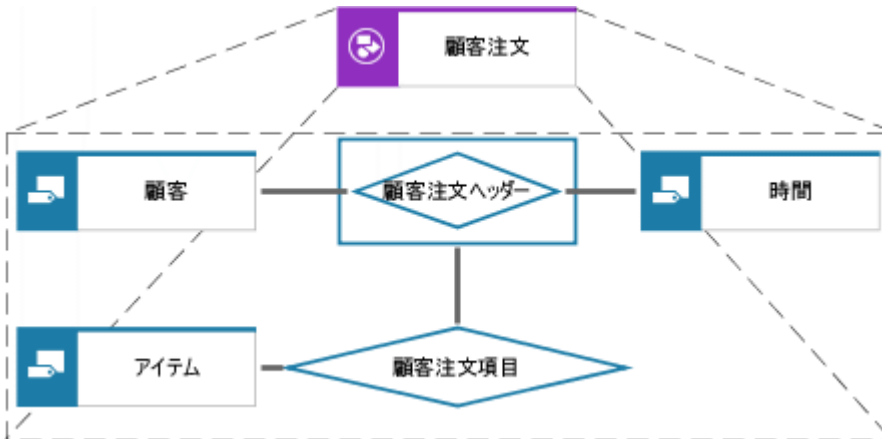
図 35: 複数のオブジェクトのデータ クラスター ビュー
