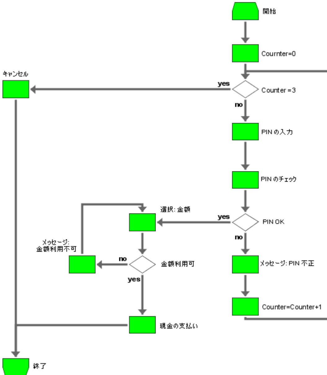
図 103: プログラム フロー図 (PF) の例
