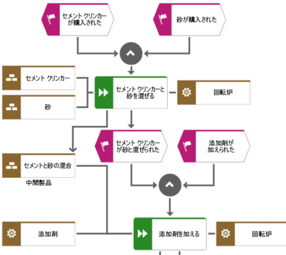
図 88: EPC (マテリアル フロー付き) からの抽出
