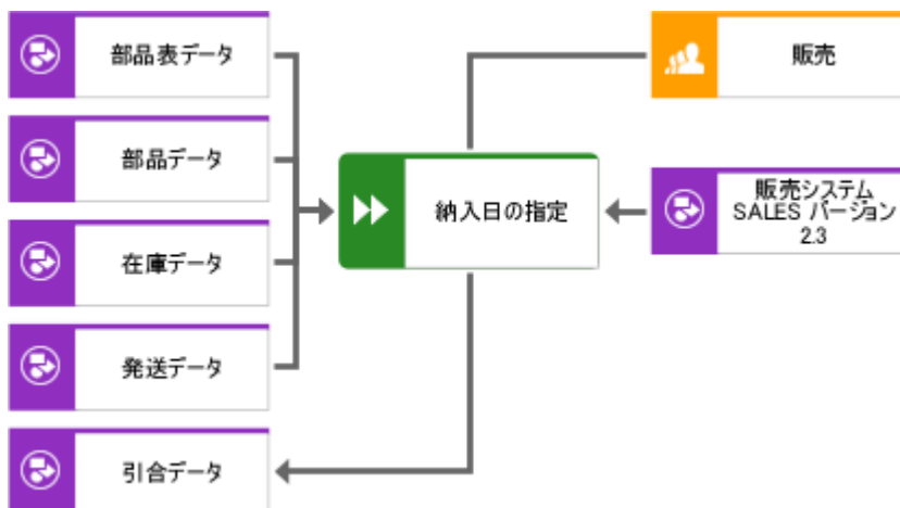
図 83: ファンクション割当図の詳細な表現
