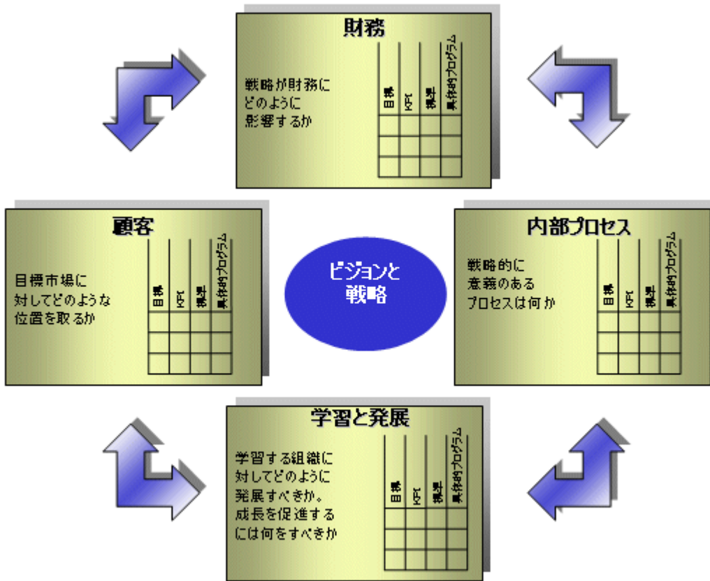
図 124: BSC の視点
