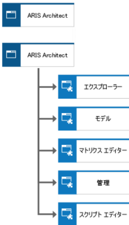
図 13: アプリケーション システム タイプのモジュール構造
