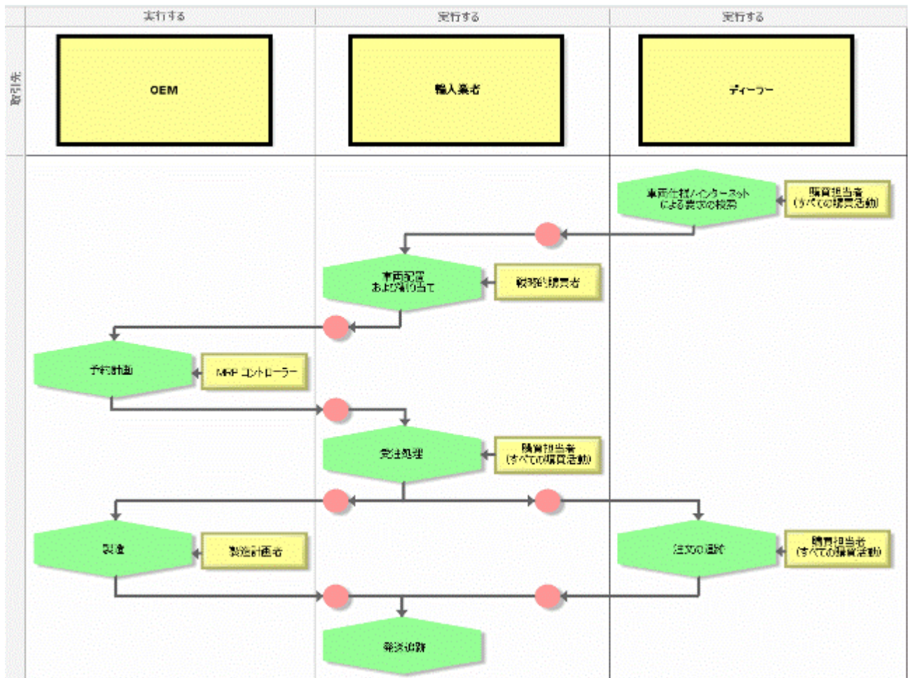
図 91: 自動車業界の e-ビジネス シナリオ図の例
