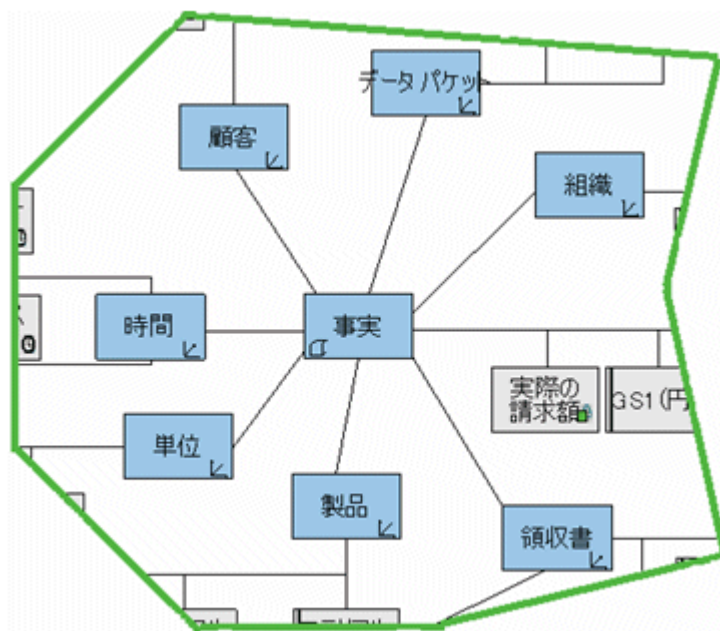
図 48: スター スキーマの Data Warehouse
