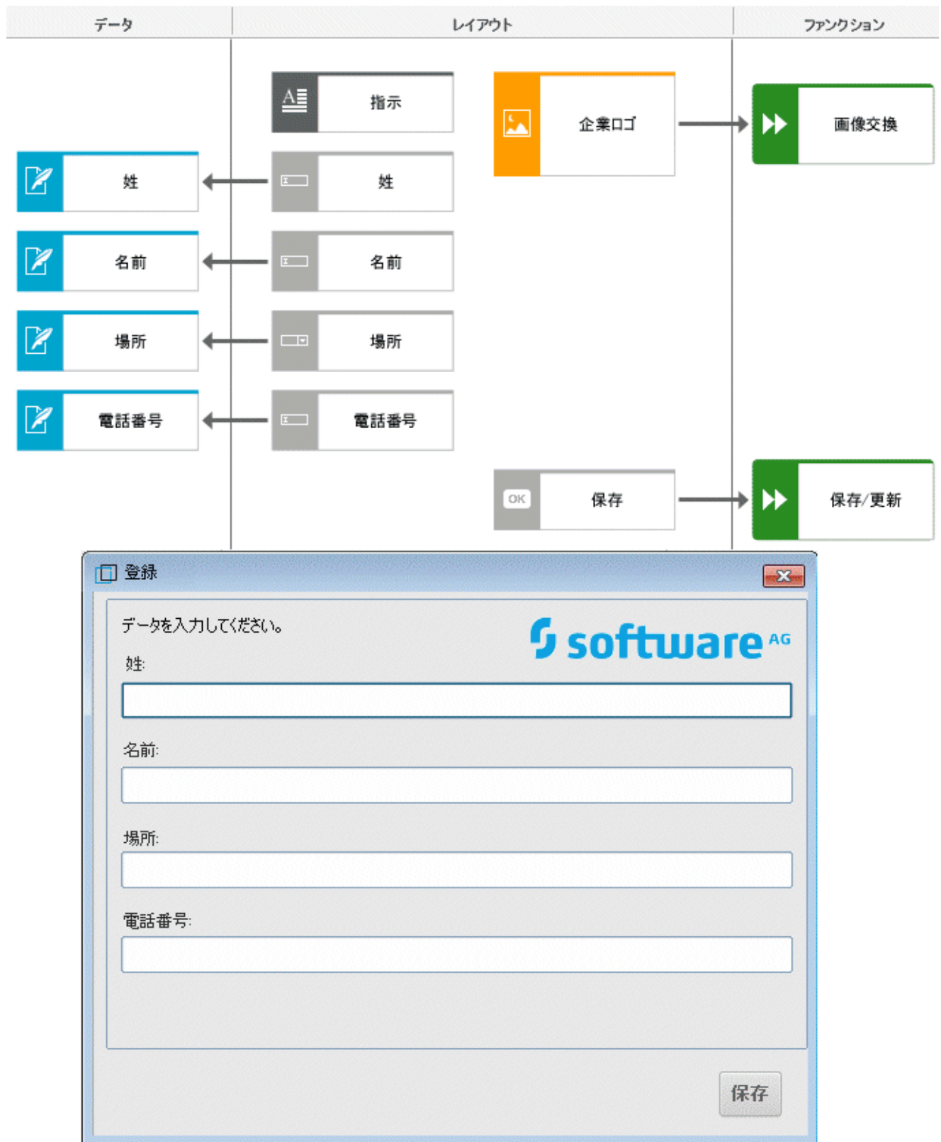
図 94: 登録ダイアログの画面設計と C++ での実装の例
