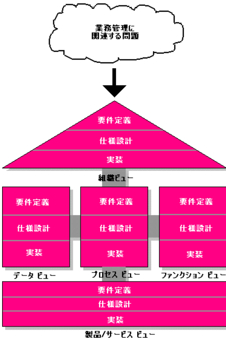
図 5: ARIS の概念
