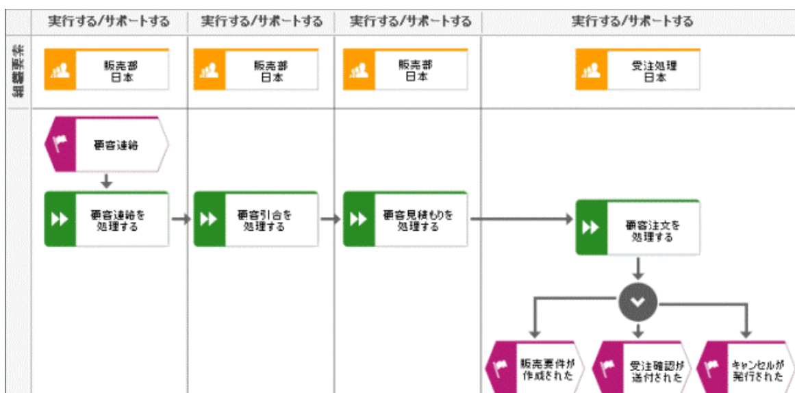
図 89: EPC (列表示)
