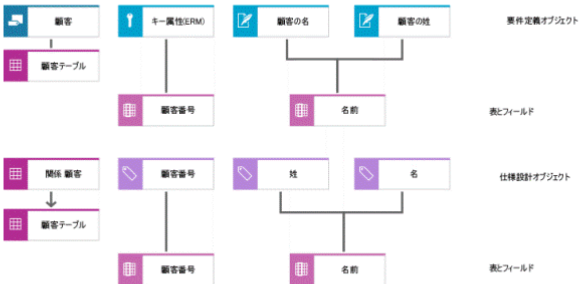
図 52: 要件定義および設計仕様オブジェクトの割り当て
