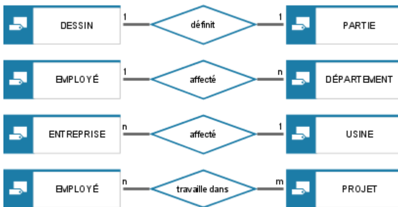
Illustration 29: Représentation des cardinalités dans MER
