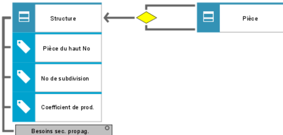
Illustration 160: Modélisation d'une association sous forme de classe
