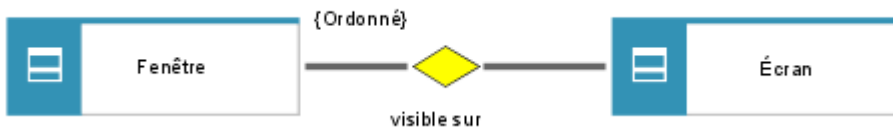
Illustration 162: Représentation d'ordres dans les associations
