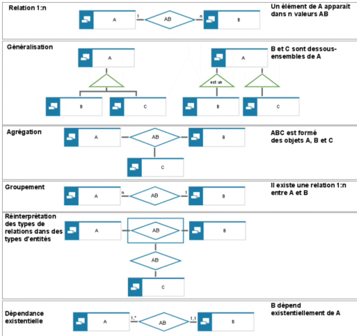
Illustration 52: Termes et formes de représentations du MERe
