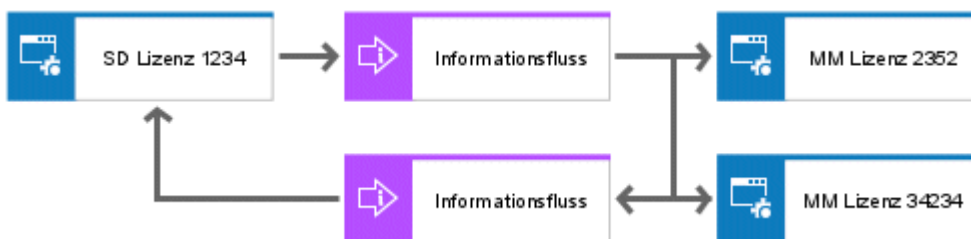
Abbildung 106: Datenfluss
