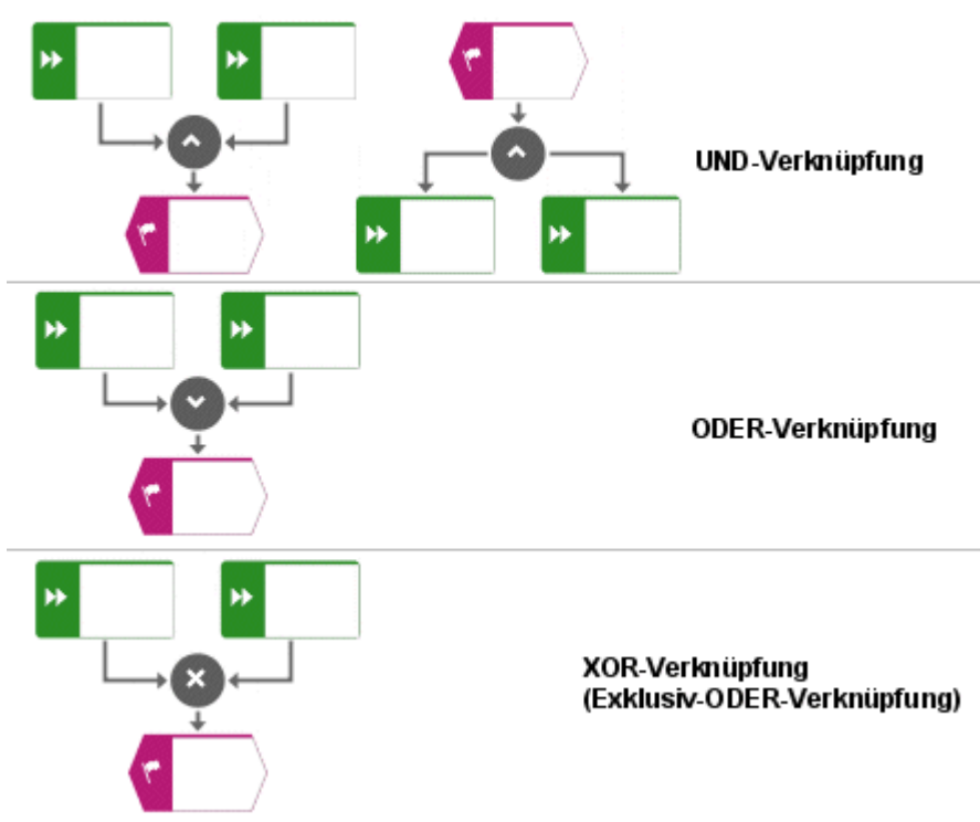
Abbildung 71: Verknüpfungsoperatoren (Regeln)
