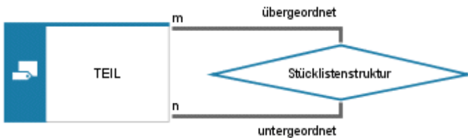
Abbildung 27: ERM für eine Stückliste
