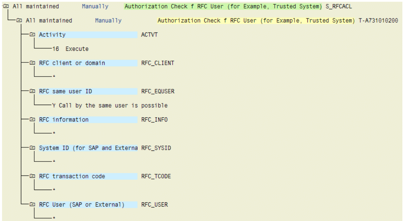
図 7: 「S_RFCACL」認証オブジェクト
