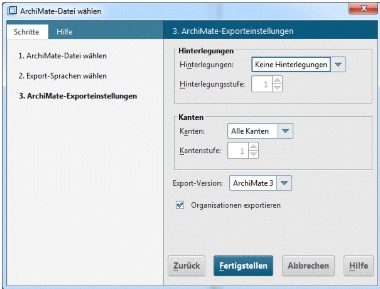
Abbildung 5: ArchiMate®-Exporteinstellungen
