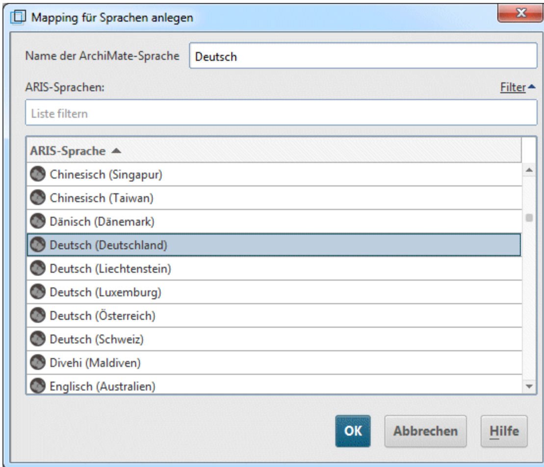
Abbildung 7: ArchiMate®-Sprach-Mapping
