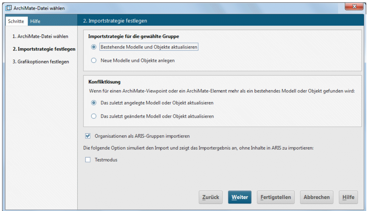
Abbildung 1: ArchiMate®-Importstrategie
