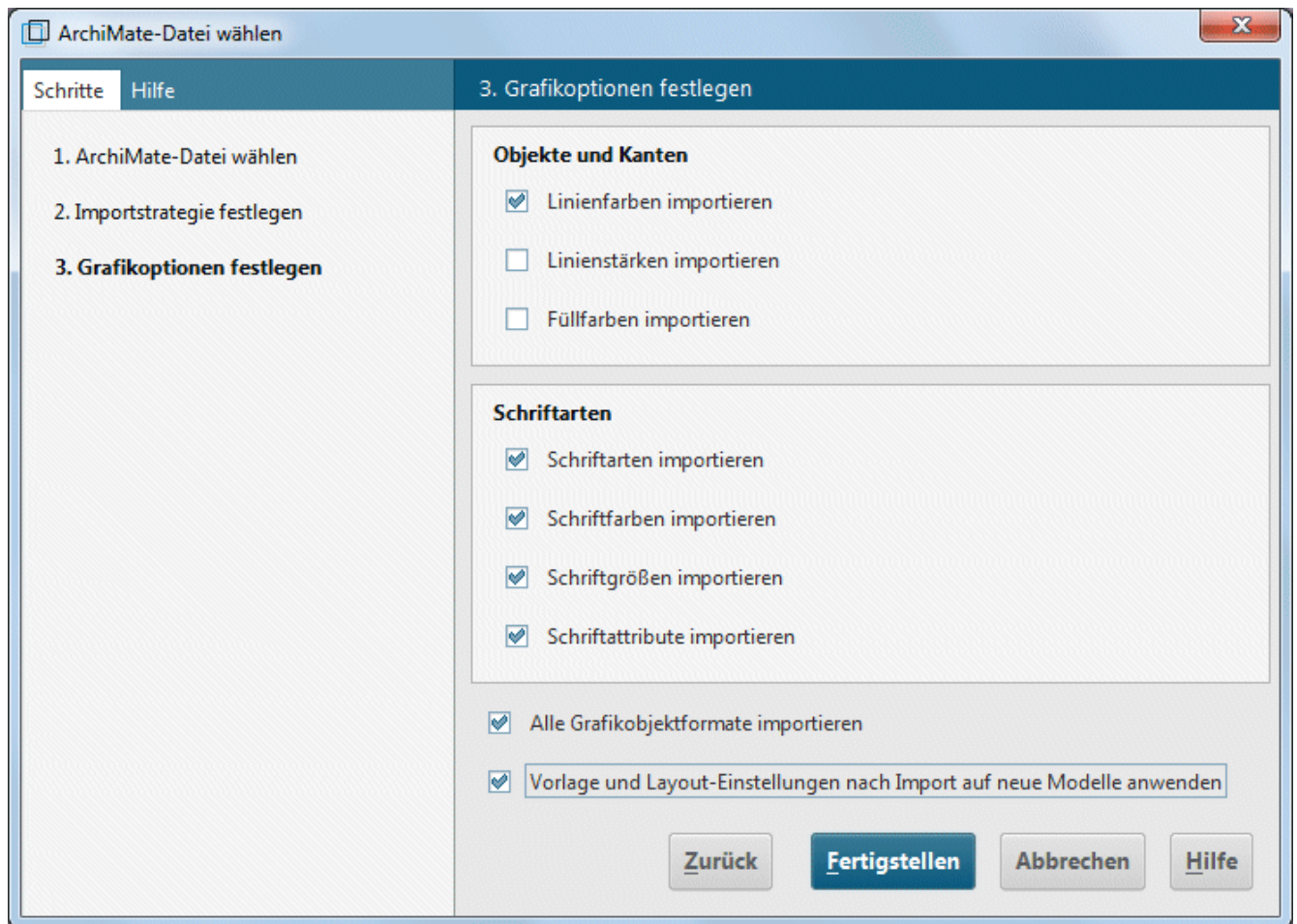
Abbildung 2: ArchiMate®-Importeinstellungen
