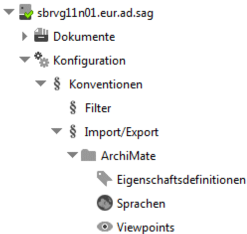
Abbildung 6: ArchiMate®-Mapping-Optionen
