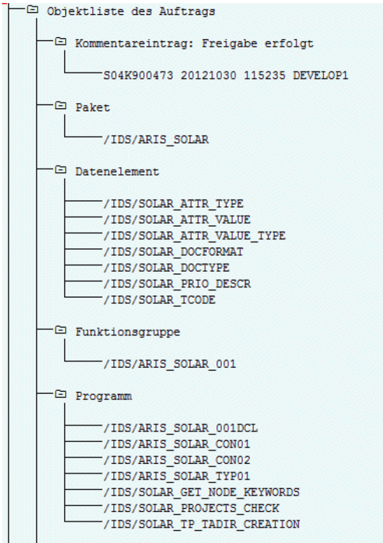
Abbildung 3: Transportauftrag: SAP®-Synchronisation (1)
