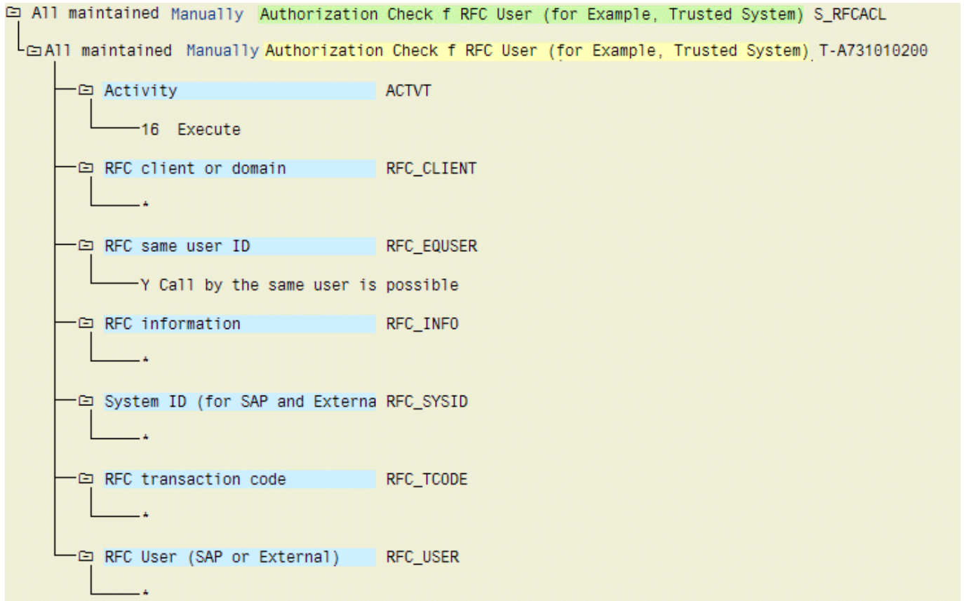
Abbildung 7: Berechtigungsobjekt 'S_RFCACL'
