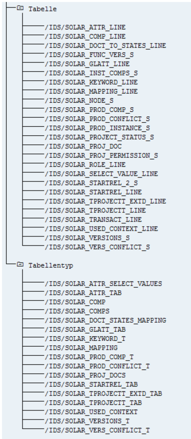
Abbildung 4: Transportauftrag: SAP®-Synchronisation (2)
