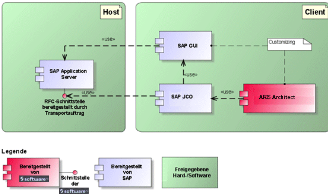
Abbildung 2: Customizing
