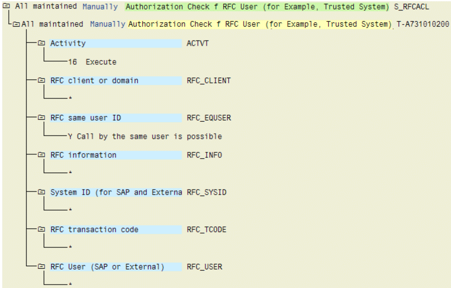
Abbildung 7: Berechtigungsobjekt 'S_RFCACL'
