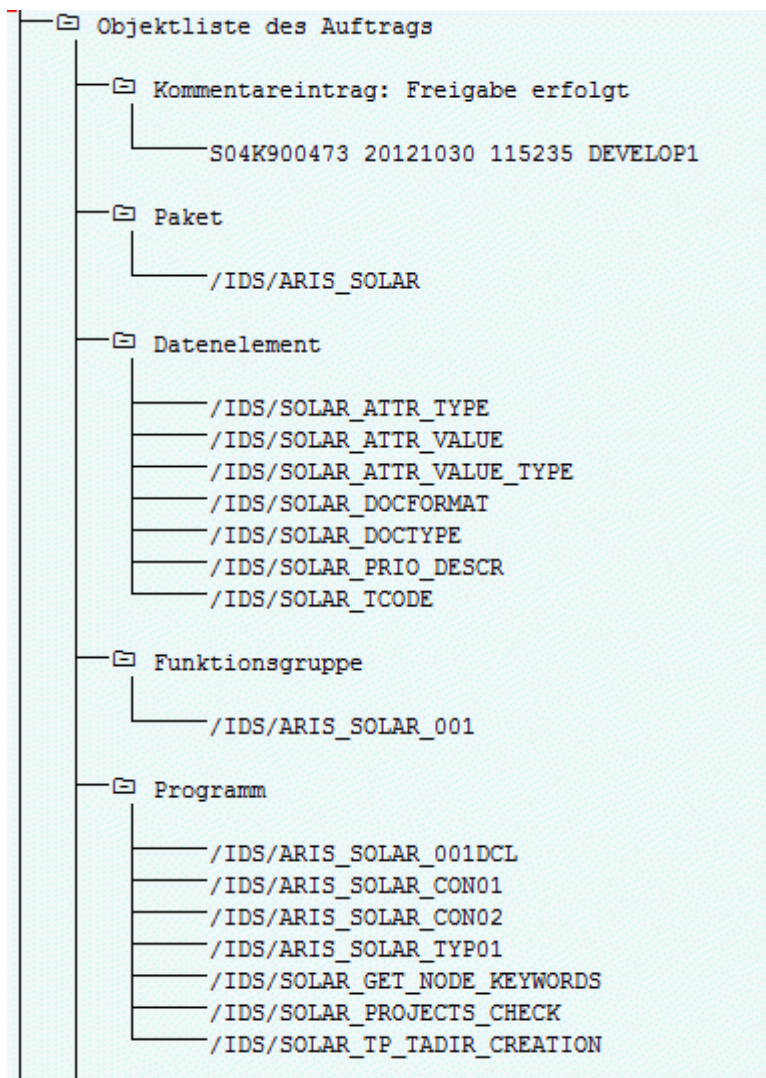
Abbildung 3: Transportauftrag: SAP®-Synchronisation (1)
