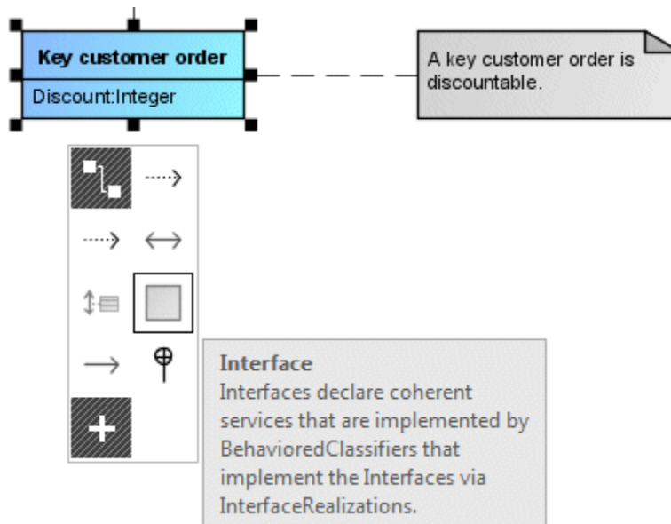
Figure 110: Mini toolbar
